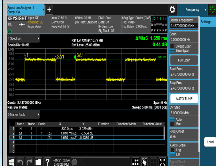
NTNV-11AX20MIMO-Ant1-2437
