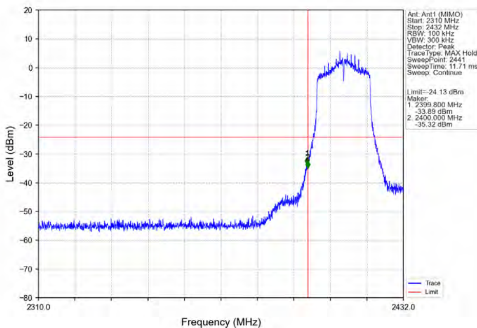
802.11ac(VHT20) LCH 2412MHz Ant1 (MIMO) NTN
