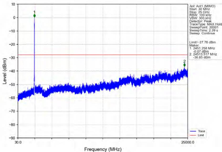
802.11ax(HEW40) HCH 2452MHz SU / Ant1 (MIMO) NTNv
