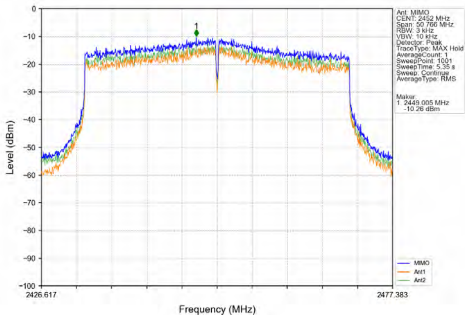
802.11ax(HEW40) HCH 2452MHz SU / MIMO NTN
