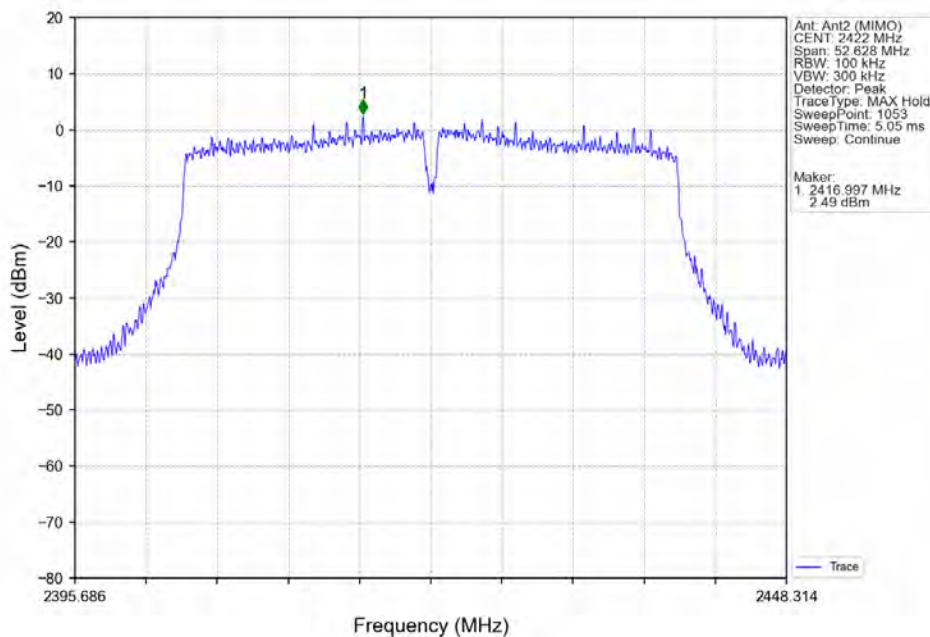
802.11n(HT40) LCH 2422MHz Ant2 (MIMO) NTN
