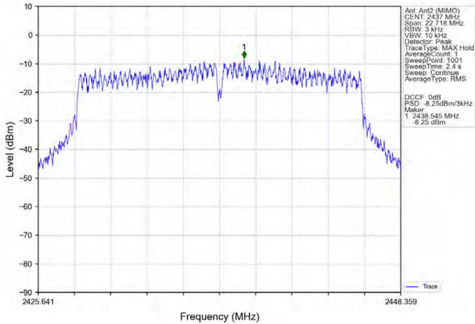
802.11ac(VHT20) MCH 2437MHz MIMO NTN
