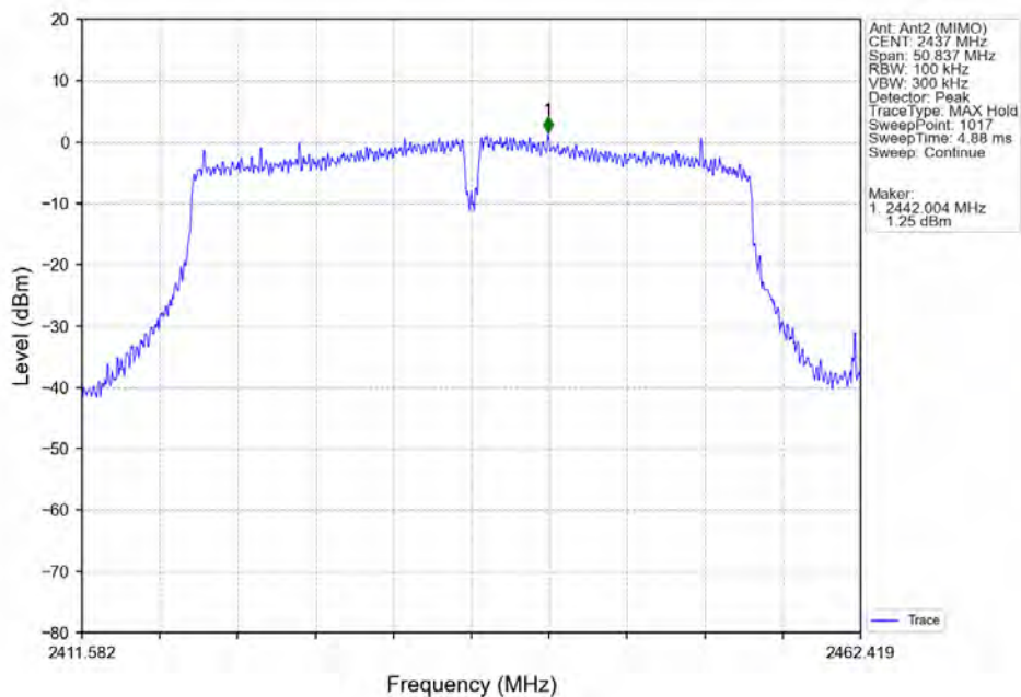
802.11n(HT40) MCH 2437MHz Ant2 (MIMO) NTV
