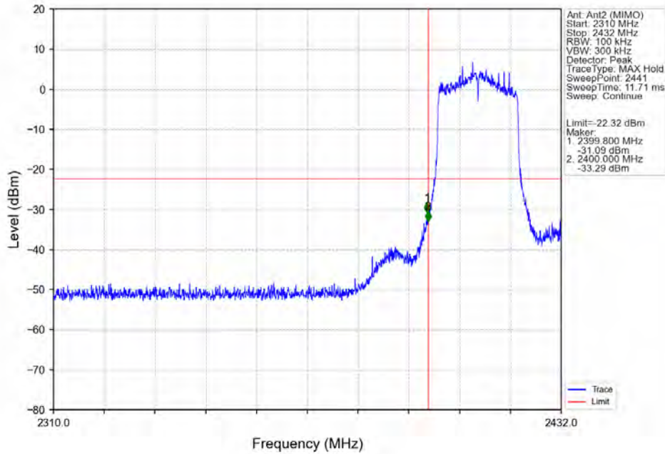
802.11ax(HEW20) LCH 2412MHz SU / Ant2 (MIMO) NTN
