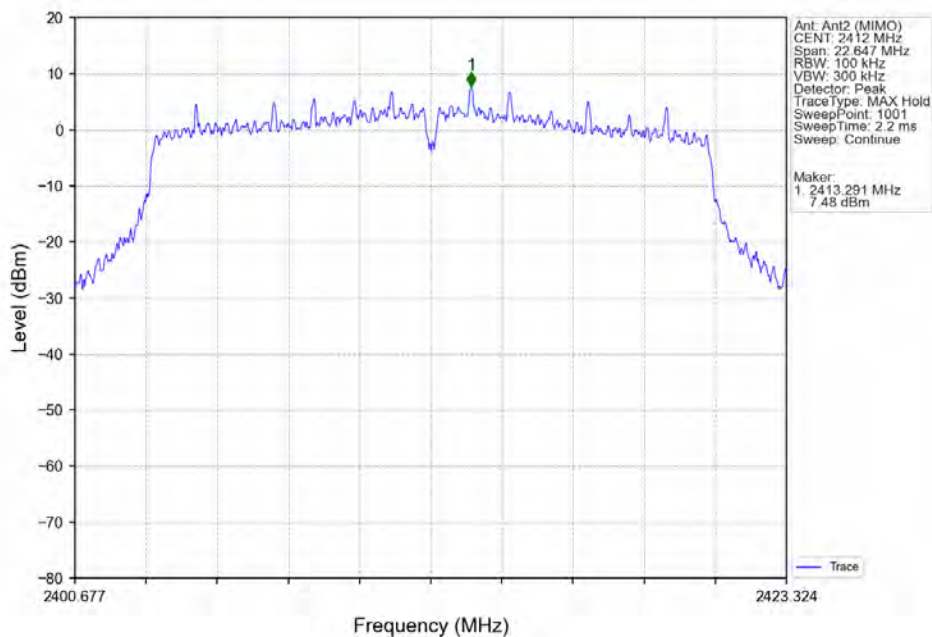
802.11ac(VHT20) LCH 2412MHz Ant2 (MIMO) NTN
