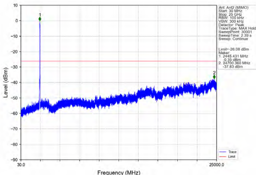
802.11ac(VHT40) HCH 2452MHz Ant2 (MIMO) NTN
