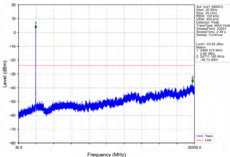
802.11n(HT20) HCH 2462MHz Ant1 (MIMO) NTN
