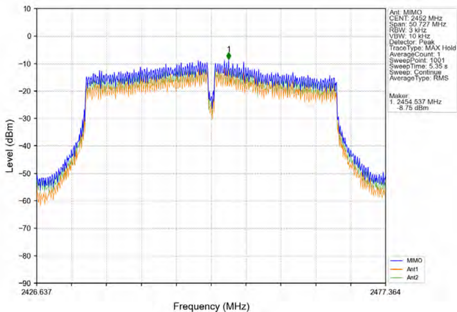
802.11ac(VHT40) HCH 2452MHz MIMO NTN
