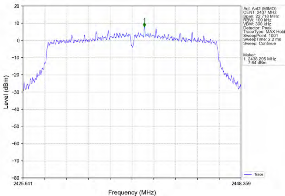
802.11ac(VHT20) MCH 2437MHz Ant2 (MIMO) NTN
