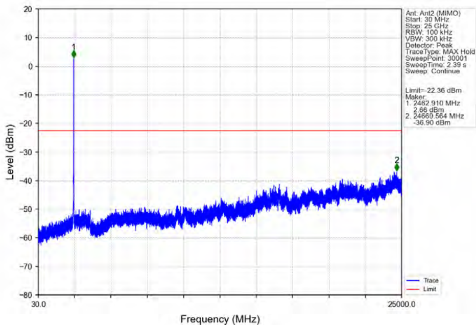
802.11ac(VHT20) HCH 2462MHz Ant2 (MIMO) NTN
