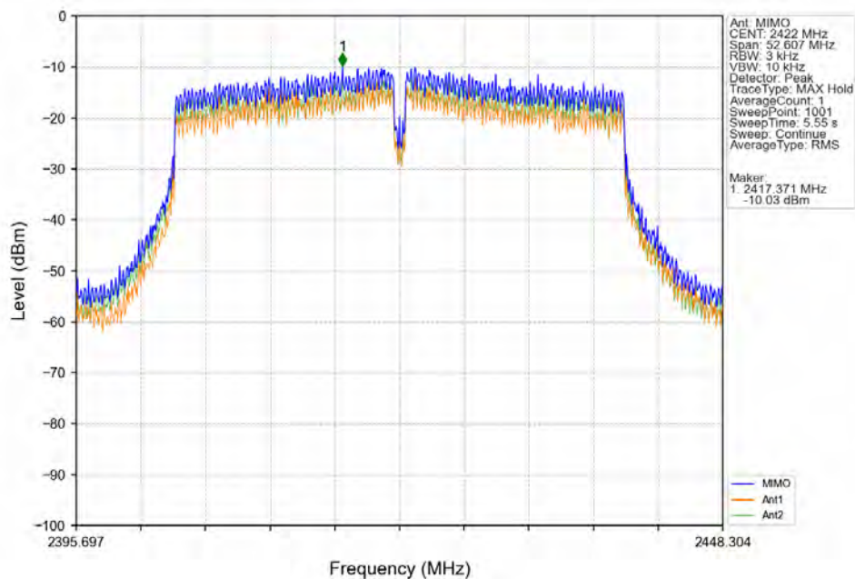
802.11ac(VHT40) LCH 2422MHz MIMO NTN
