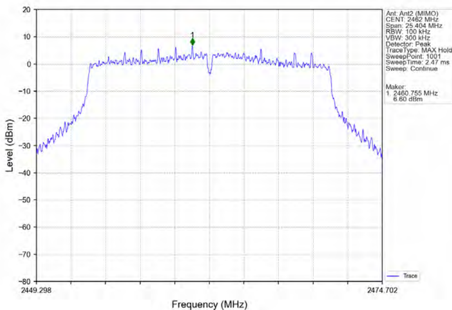
802.11n(HT20) HCH 2462MHz Ant2 (MIMO) NTVN
