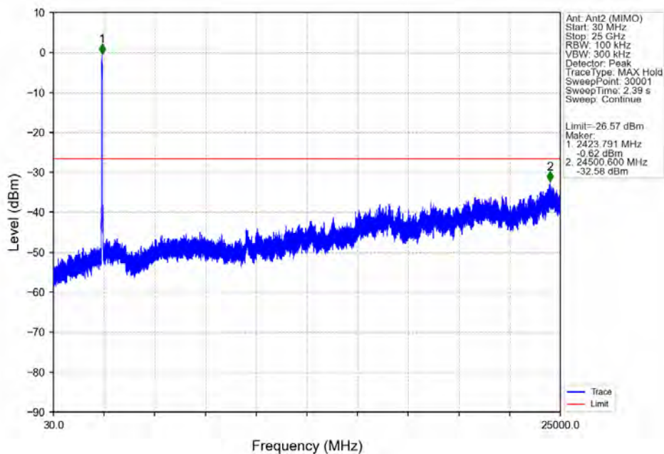
802.11ax(HEW40) LCH 2422MHz SU / Ant2 (MIMO) NTNV
