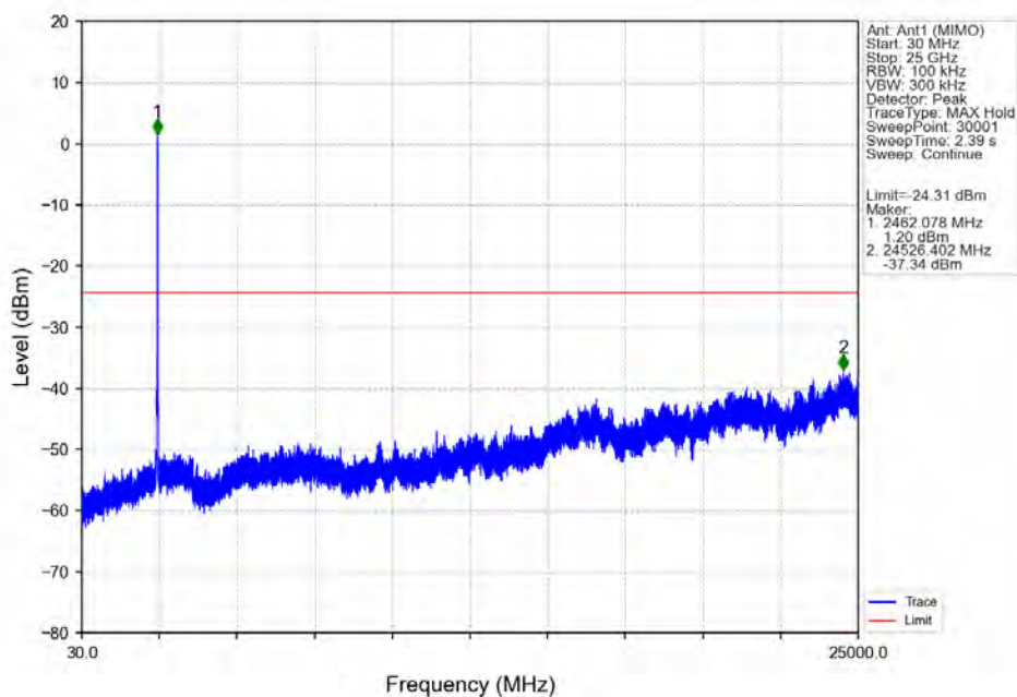
802.11ax(HEW20) HCH 2462MHz SU / Ant1 (MIMO) NTN
