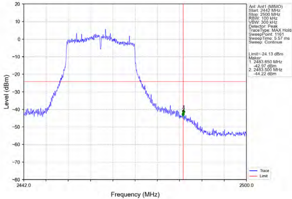
802.11ac(VHT20) HCH 2462MHz Ant1 (MIMO) NTN
