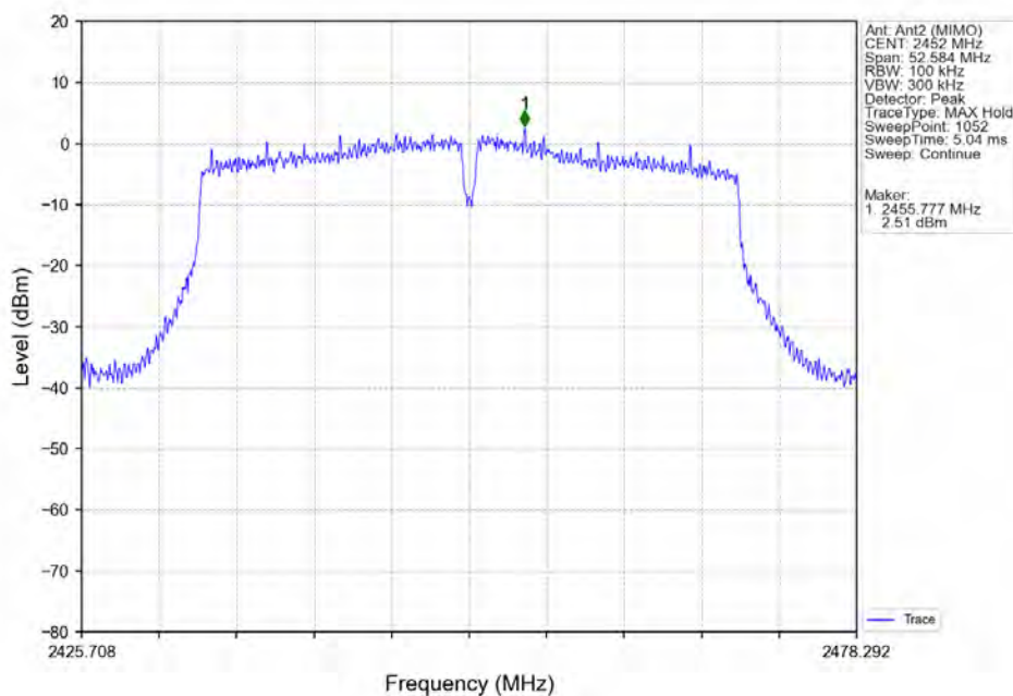
802.11n(HT40) HCH 2452MHz Ant2 (MIMO) NTVN
