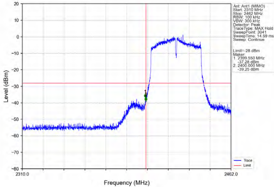
802.11ac(VHT40) LCH 2422MHz Ant1 (MIMO) NTN
