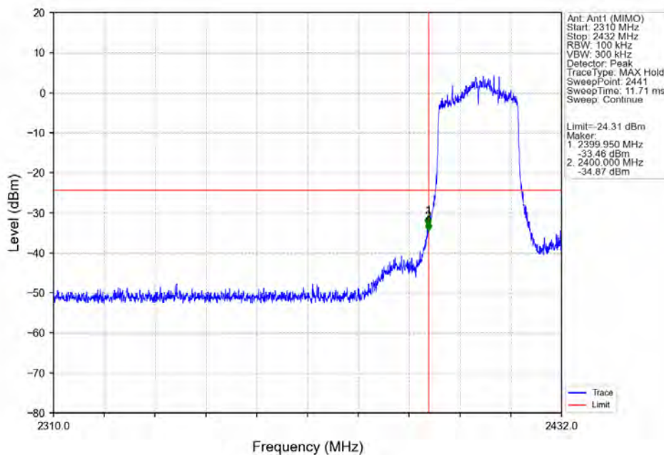
802.11ax(HEW20) LCH 2412MHz SU / Ant1 (MIMO) NTNV
