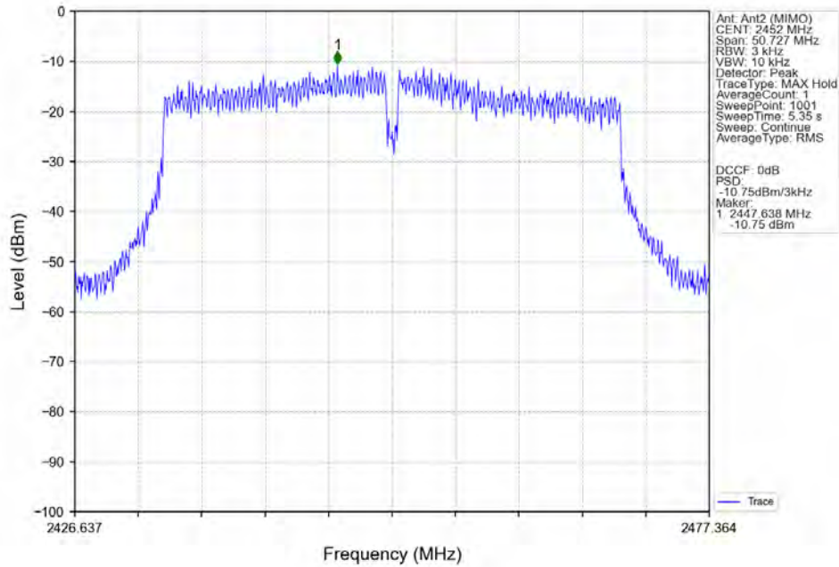
802.11ac(VHT40) HCH 2452MHz MIMO NTN
