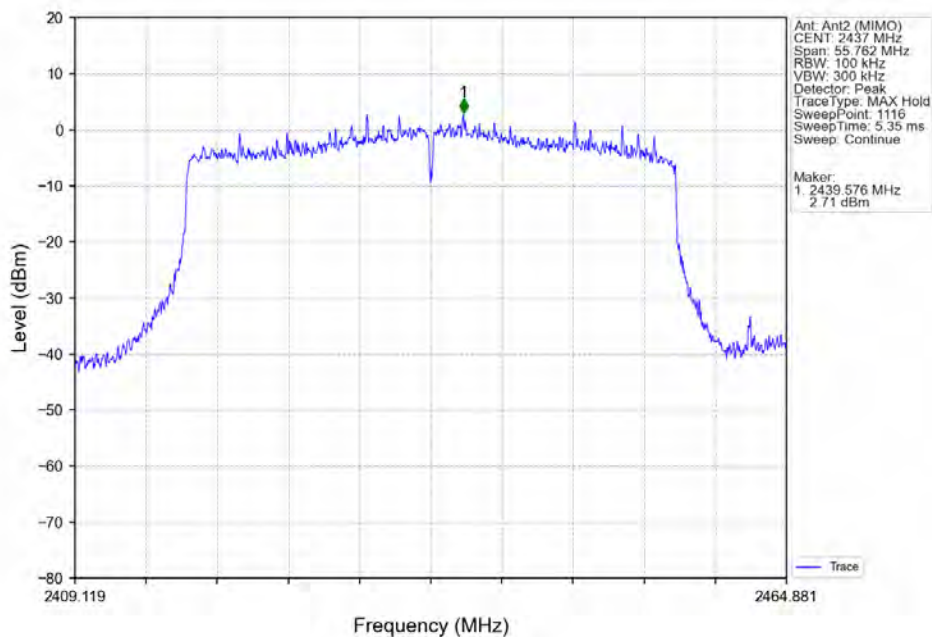
802.11ax(HEW40) MCH 2437MHz SU / Ant2 (MIMO) NTN
