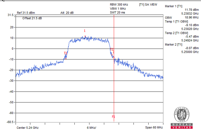
802.11ac(VHT20)_Chain1 / CH48
