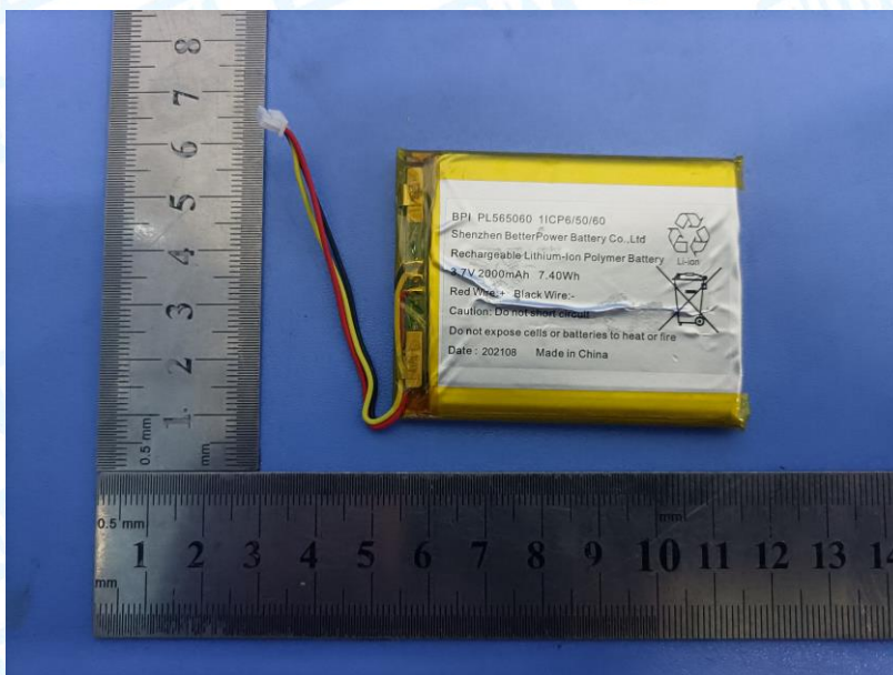
Photo 12 Battery parameters
