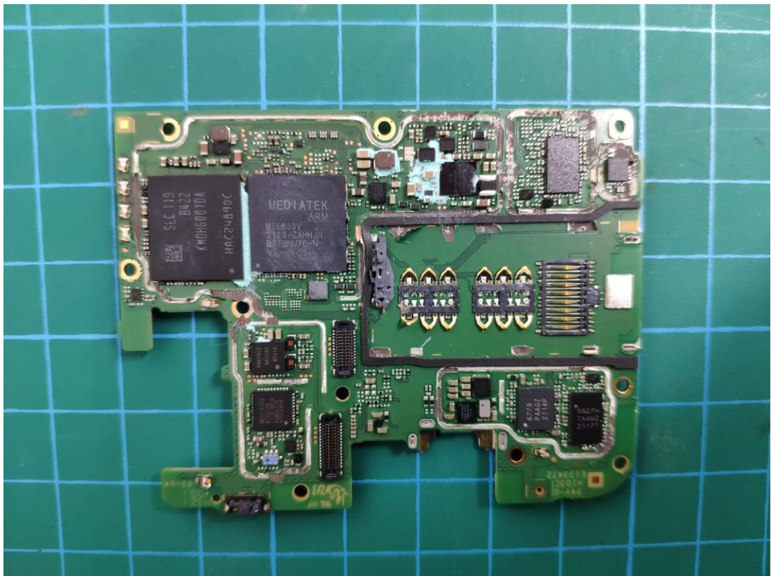
PCB 07: (NFC Chip RN82)
