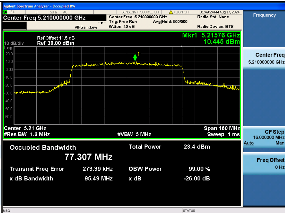
11AX80MIMO-Ant2-5210
