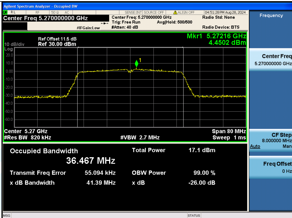
11N40MIMO-Ant3-5270
