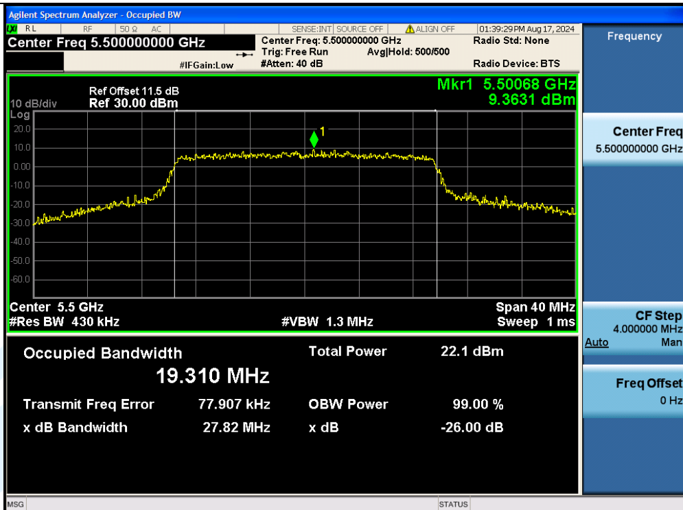
11AX20MIMO-Ant2-5500
