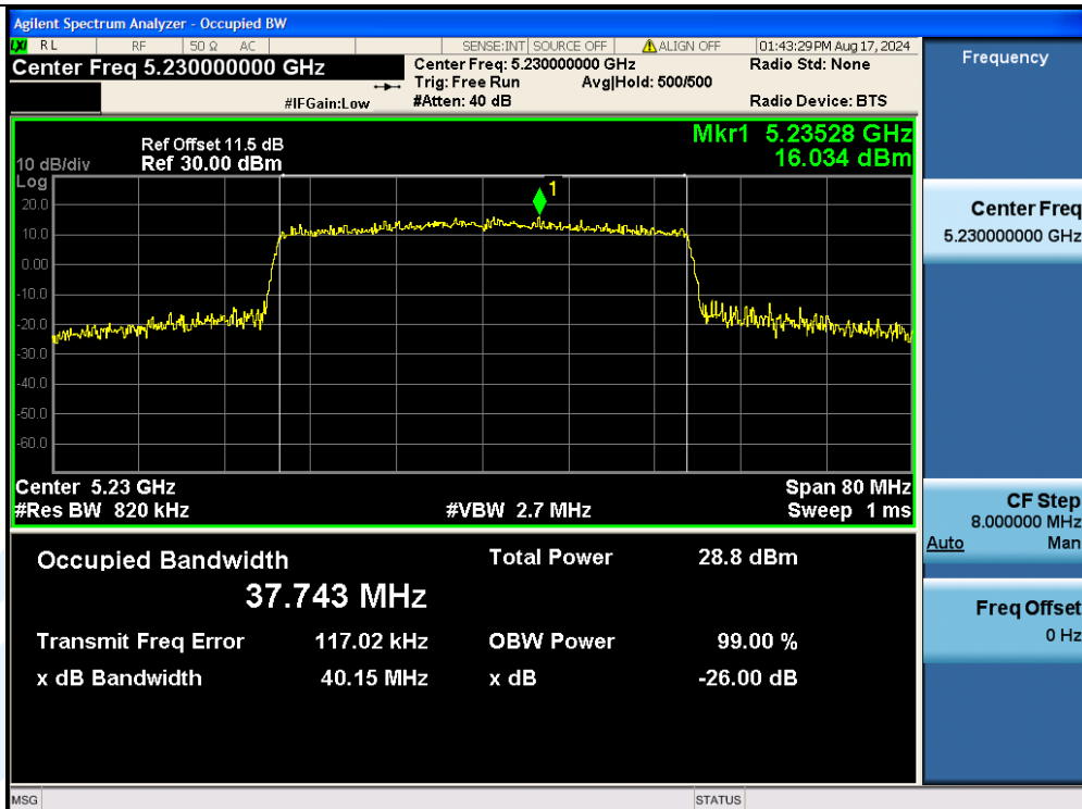
11AX40MIMO-Ant2-5230
