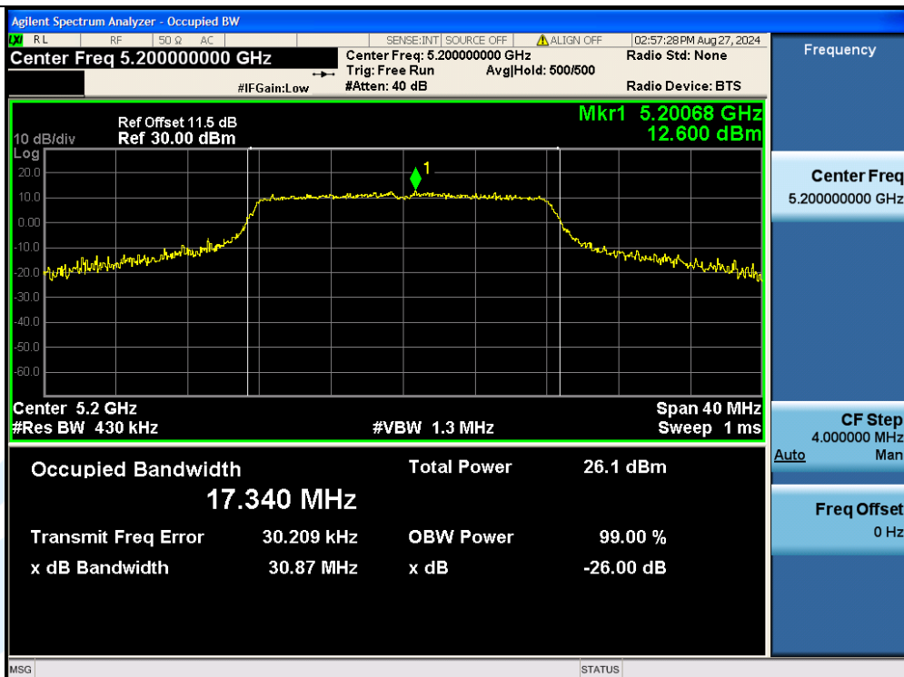
11A-Ant3-5200
