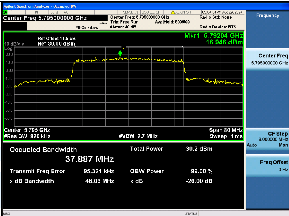
11AX40MIMO-Ant2-5795
