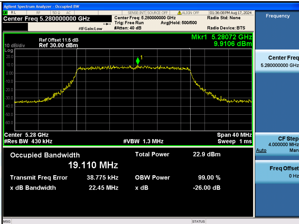
11AX20MIMO-Ant2-5280
