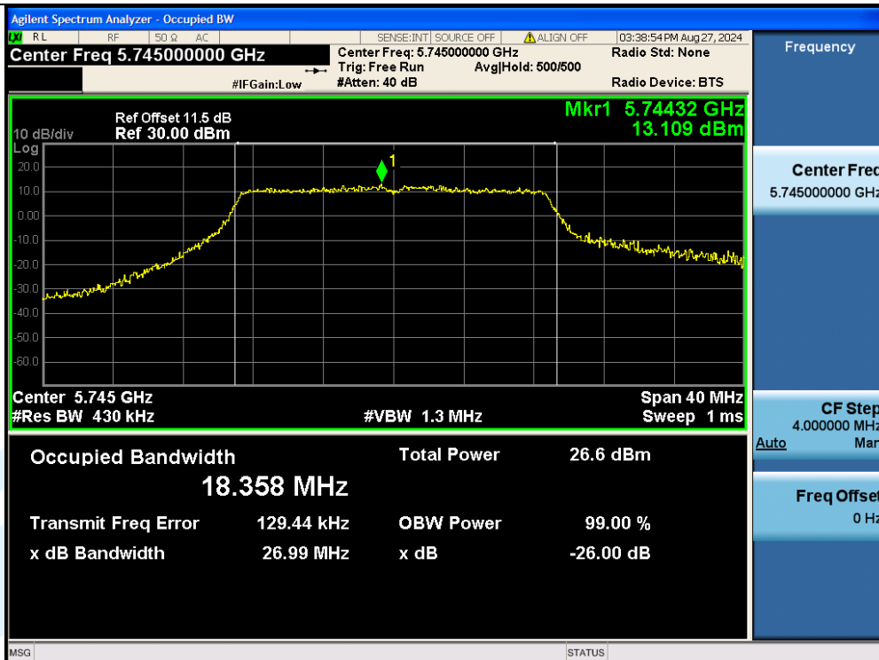
11N20MIMO-Ant3-5745
