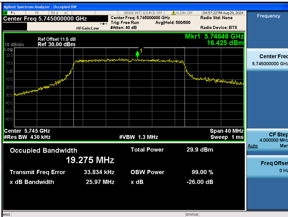
11AX20MIMO-Ant2-5745
