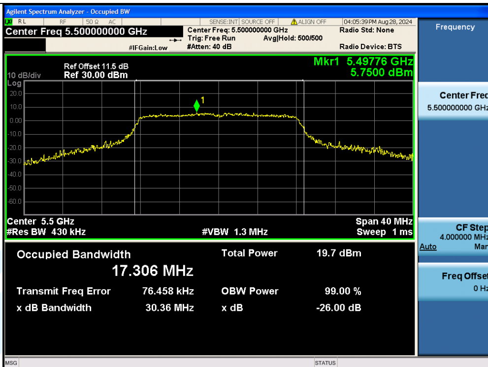
11A-Ant1-5500
