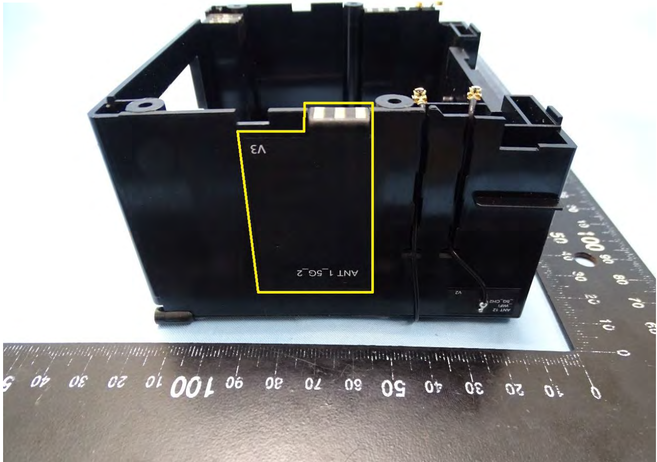
ANT 1_WWAN Antenna
