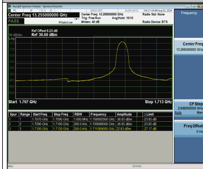
Band66_20MHz_QPSK_132072_1RB#0
