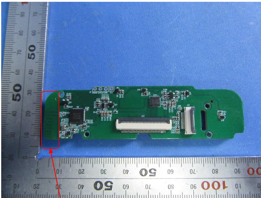
BLE antenna
