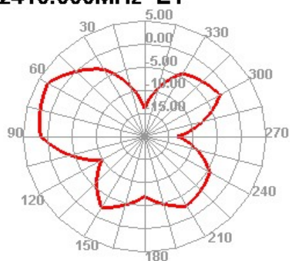
2410.000MHz E1
