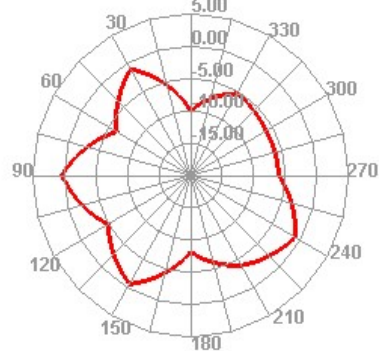
5160.000MHz H
