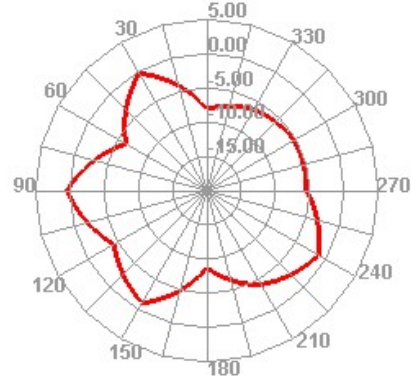
5160.000MHz E2
