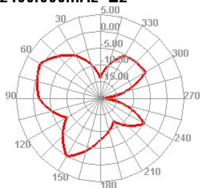
2410.000MHz H
