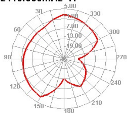
2410.000MHz H
