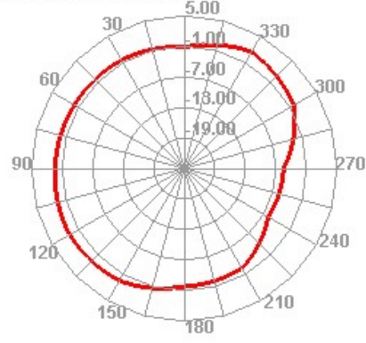
5160.000MHz E2
