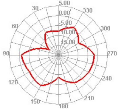
5160.000MHz E1
