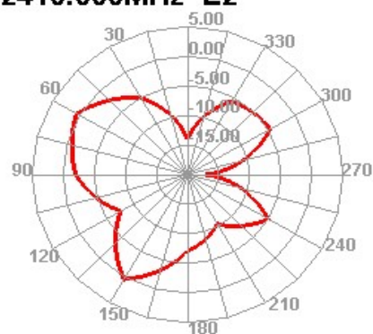
2410.000MHz E2
