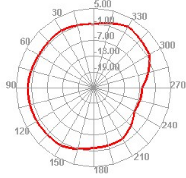
5150.000MHz E2
