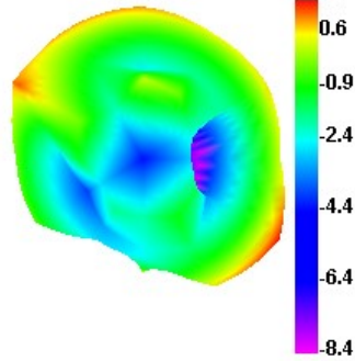
5150.000MHz E1
