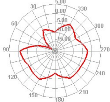
5160.000MHz
