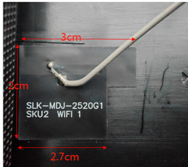
BT/WIFI ANT
