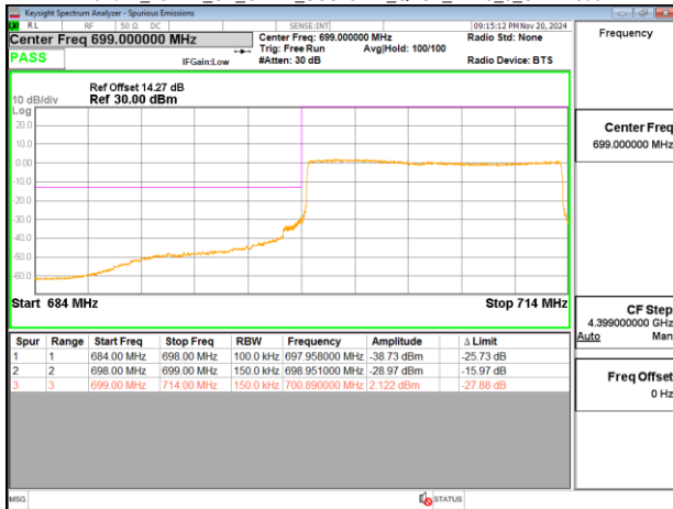
Band12_15MHz_CP_OFDM_SCS15kHz_QPSK_RB1_78_CH141700
