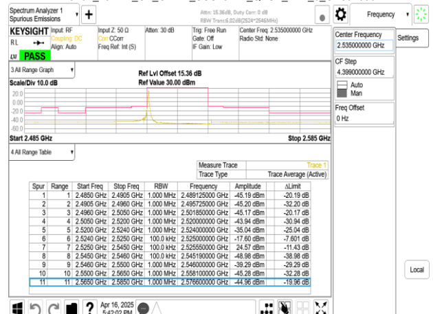
Band7_20MHz_CP_OFDM_SCS15kHz_QPSK_RB1_0_CH507000
