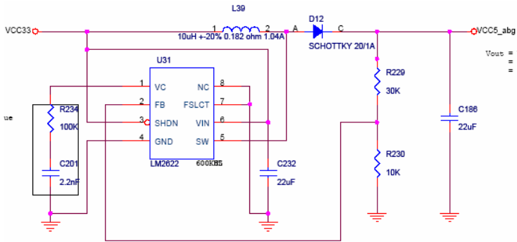
圖二 PA 5V 電壓產生電路圖
