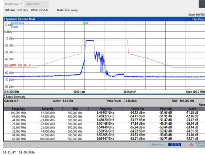
11AX40MIMO_Ant1_6525_242Tone_RU61
