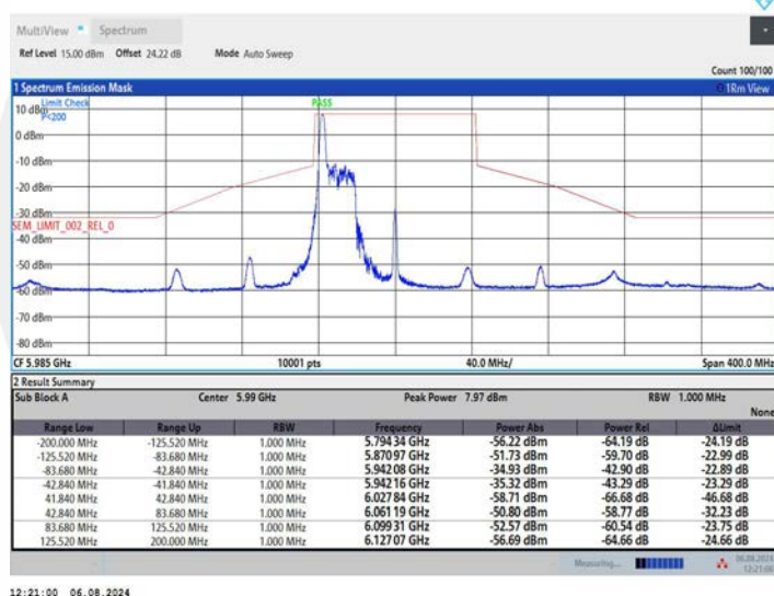
11AX80MIMO_Ant2_5985_52Tone_RU37
