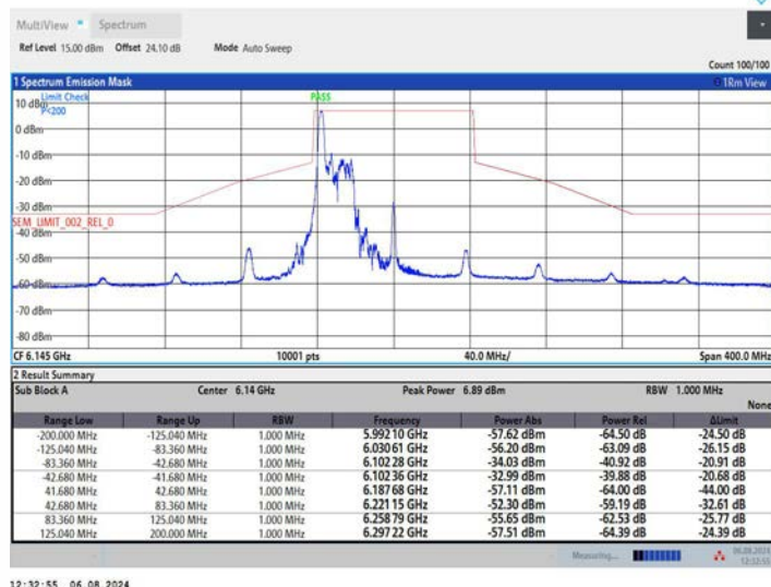
11AX80MIMO_Ant1_6145_52Tone_RU37
