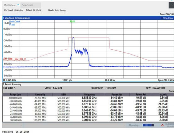
11AX40MIMO_Ant2_6925_52Tone_RU37
