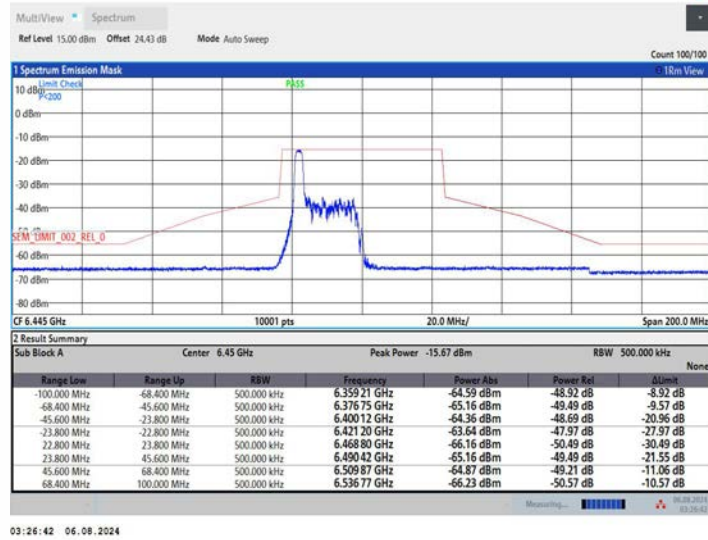
11AX40MIMO_Ant2_6445_52Tone_RU37
