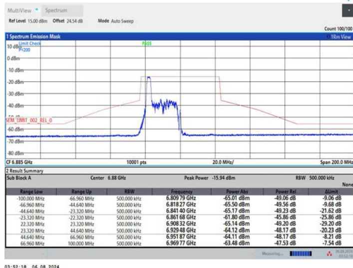
11AX40MIMO_Ant2_6885_52Tone_RU37
