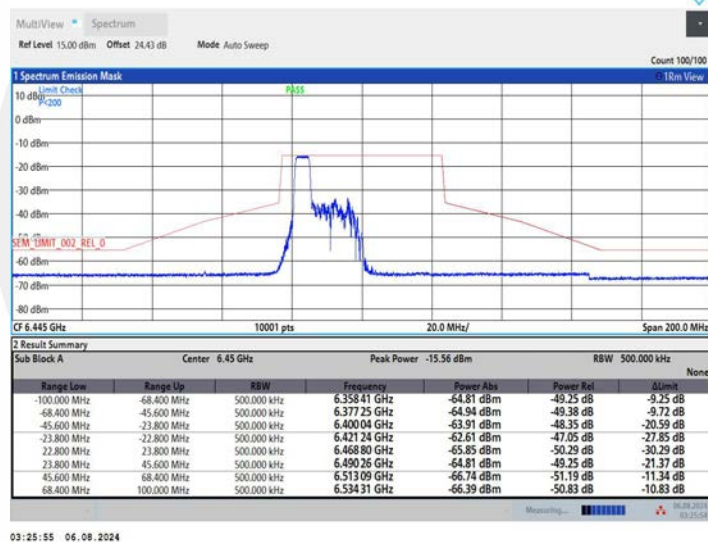
11AX40MIMO_Ant2_6445_106Tone_RU53
