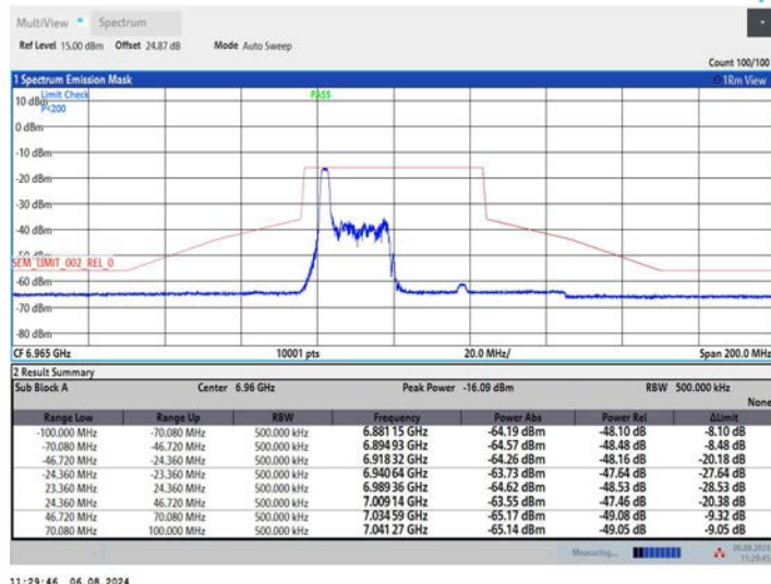
11AX40MIMO_Ant2_6965_52Tone_RU37
