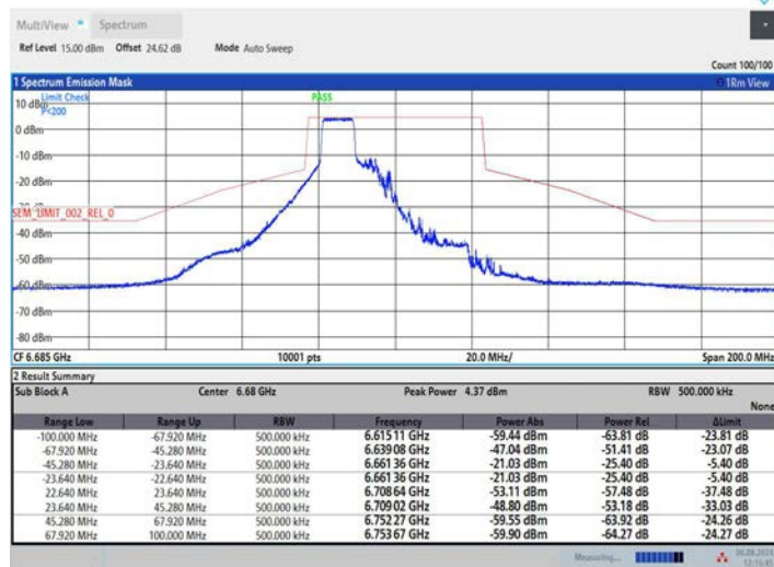
11AX40MIMO_Ant2_6685_242Tone_RU61
