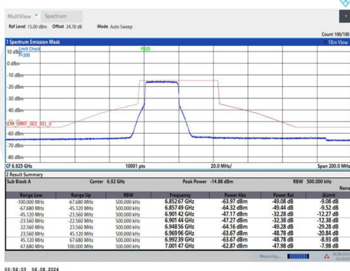
11AX40MIMO_Ant2_6925_26Tone_RU0
