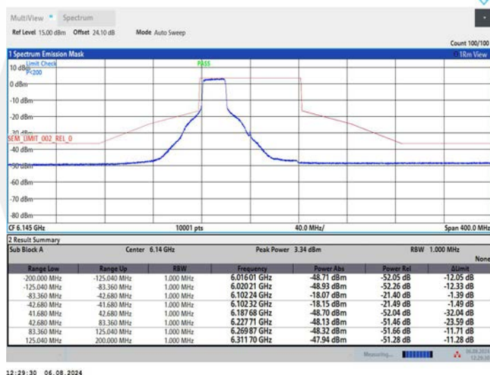
11AX80MIMO_Ant1_6145_484Tone_RU65
