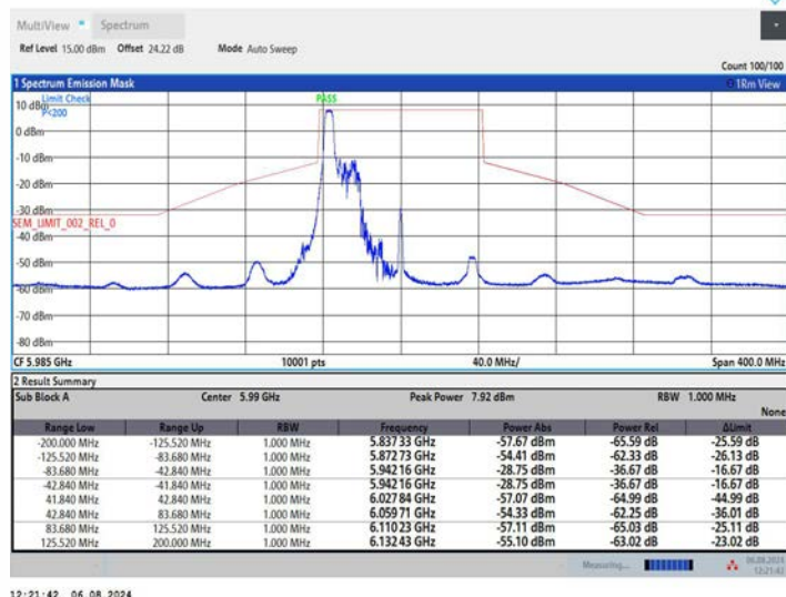
11AX80MIMO_Ant2_5985_106Tone_RU53
