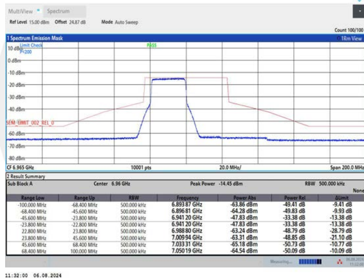
11AX40MIMO_Ant2_6965_26Tone_RU0
