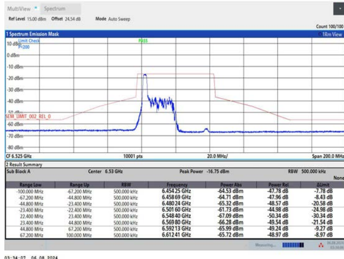
11AX40MIMO_Ant1_6525_52Tone_RU37
