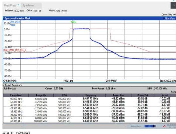
11AX40MIMO_Ant2_6565_26Tone_RU0
