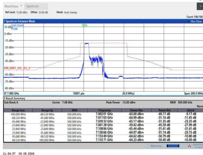
11AX40MIMO_Ant1_7085_106Tone_RU53
