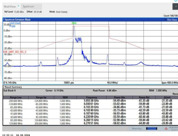
11AX80MIMO_Ant2_6145_52Tone_RU37
