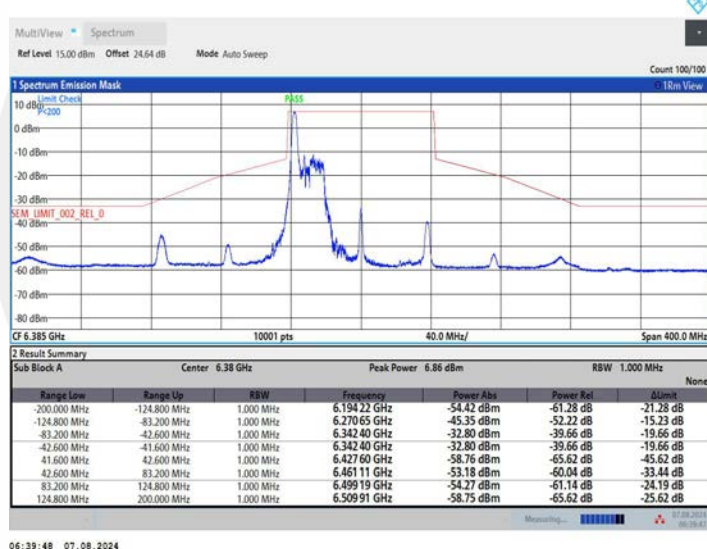
11AX80MIMO_Ant2_6385_52Tone_RU37
