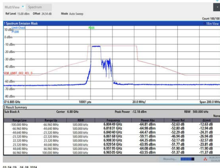
11AX40MIMO_Ant2_6885_242Tone_RU61
