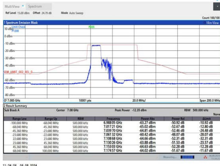
11AX40MIMO_Ant2_7085_242Tone_RU61
