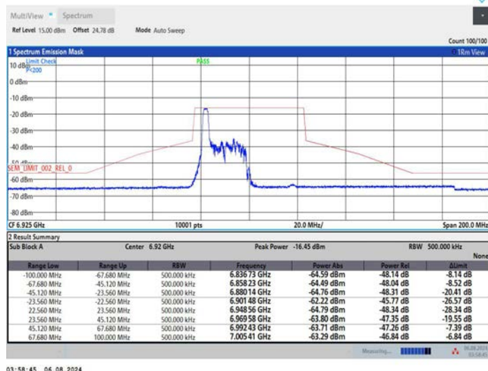
11AX40MIMO_Ant1_6925_52Tone_RU37
