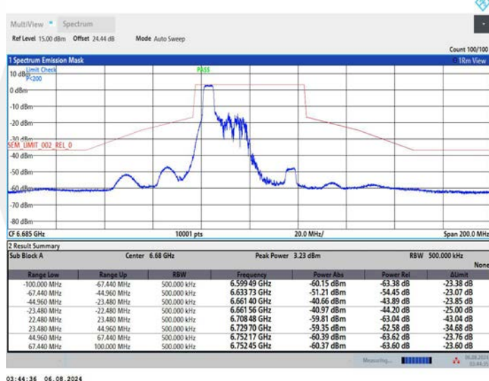
11AX40MIMO_Ant1_6685_106Tone_RU53
