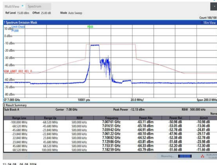
11AX40MIMO_Ant1_7085_242Tone_RU61
