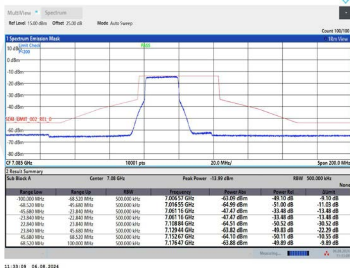
11AX40MIMO_Ant2_7085_26Tone_RU0
