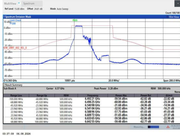
11AX40MIMO_Ant1_6565_242Tone_RU61
