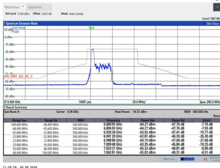
11AX40MIMO_Ant1_6965_52Tone_RU37
