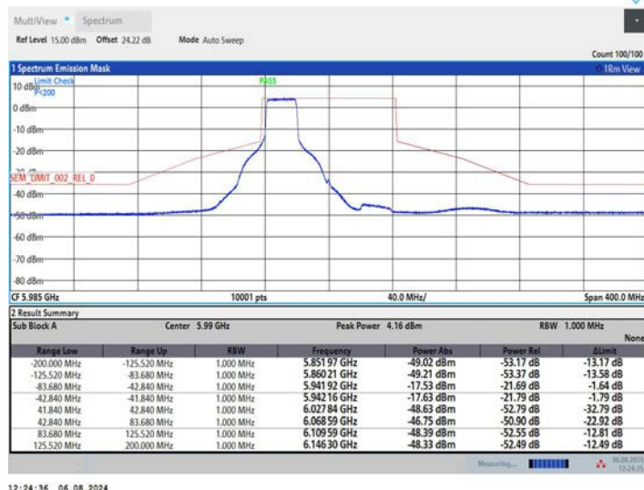
11AX80MIMO_Ant2_5985_484Tone_RU65
