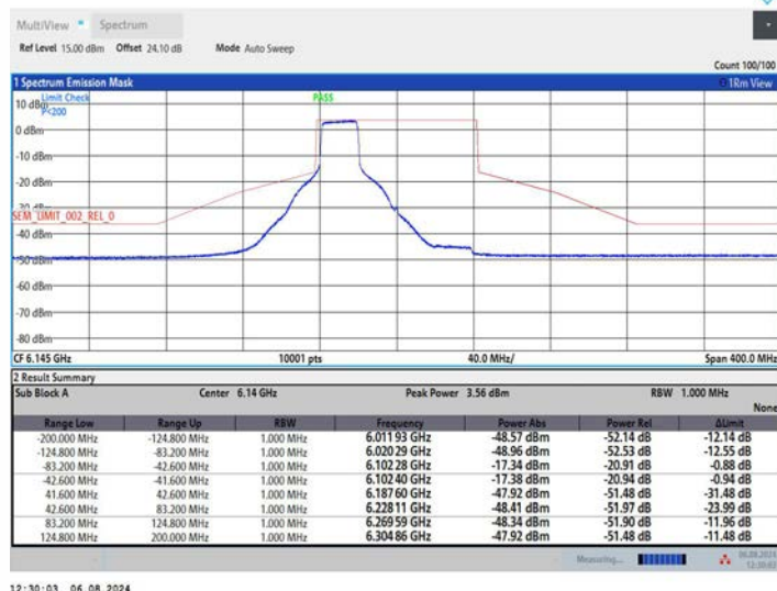
11AX80MIMO_Ant2_6145_484Tone_RU65
