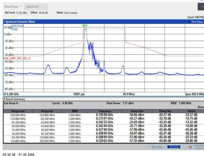
11AX80MIMO_Ant2_6385_106Tone_RU53
