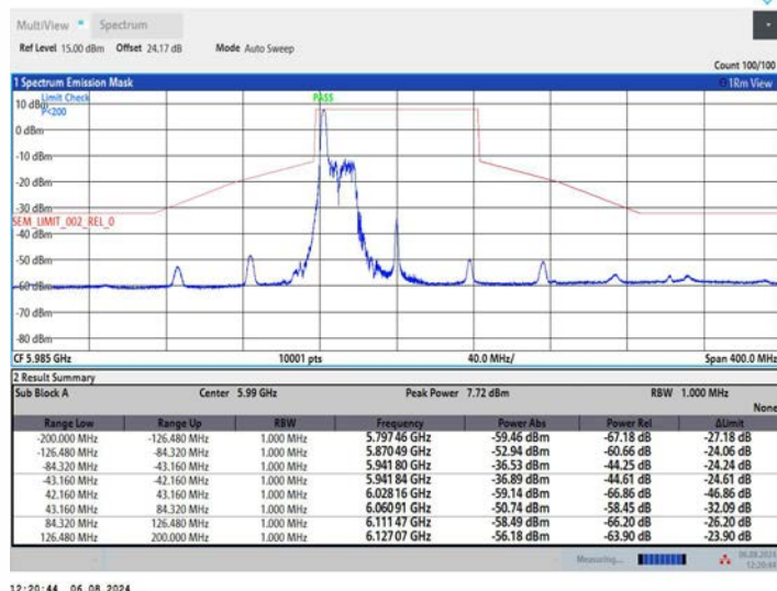
11AX80MIMO_Ant1_5985_52Tone_RU37
