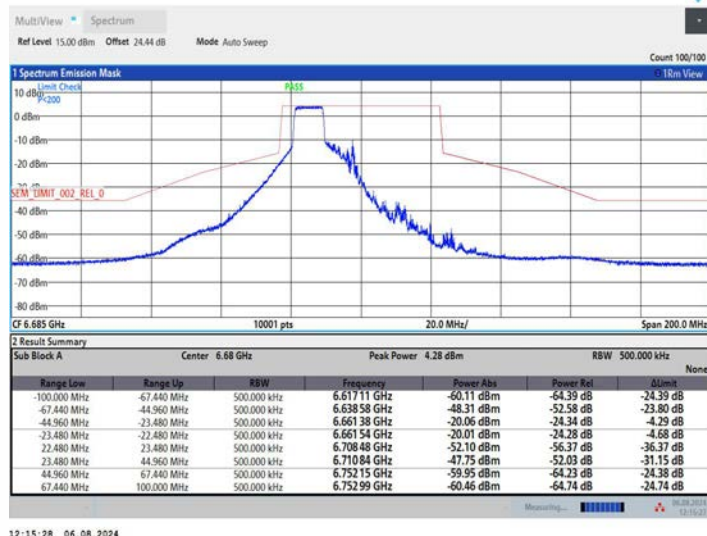
11AX40MIMO_Ant1_6685_242Tone_RU61
