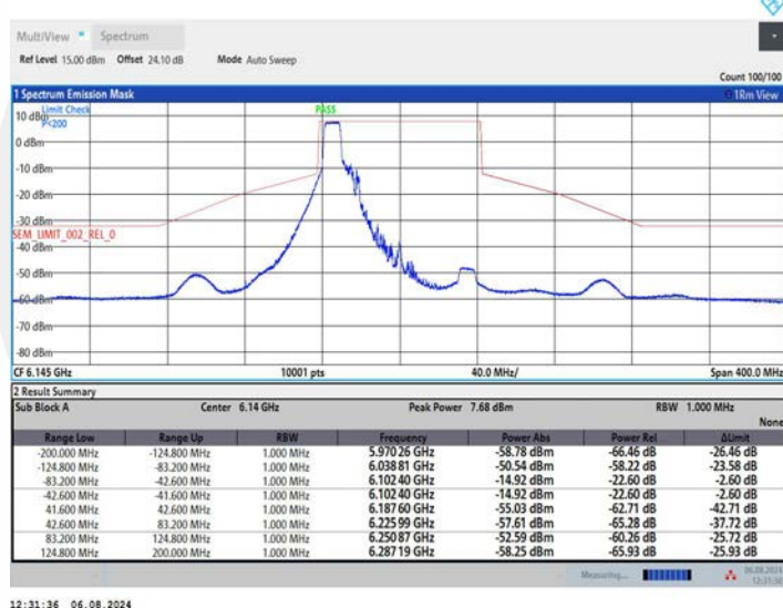
11AX80MIMO_Ant2_6145_242Tone_RU61
