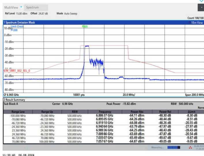
11AX40MIMO_Ant2_6965_106Tone_RU53
