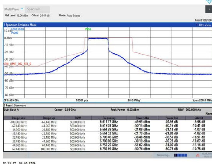
11AX40MIMO_Ant2_6685_26Tone_RU0
