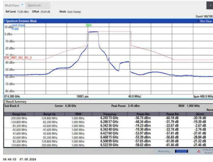
11AX80MIMO_Ant2_6385_484Tone_RU65
