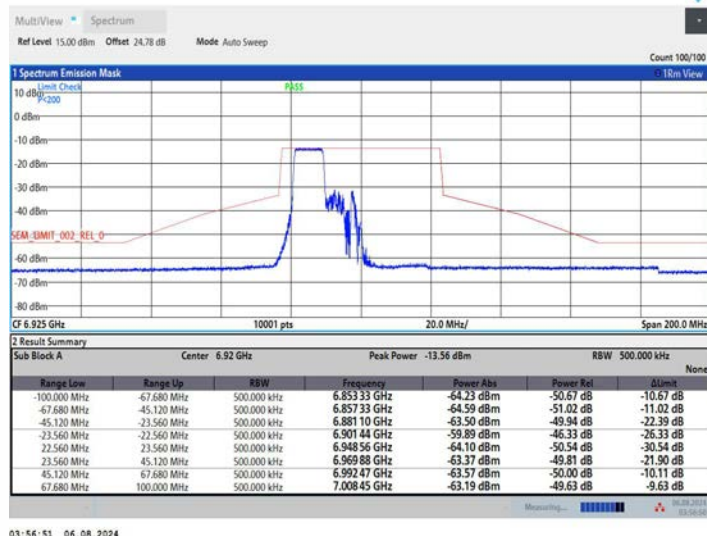
11AX40MIMO_Ant1_6925_242Tone_RU61
