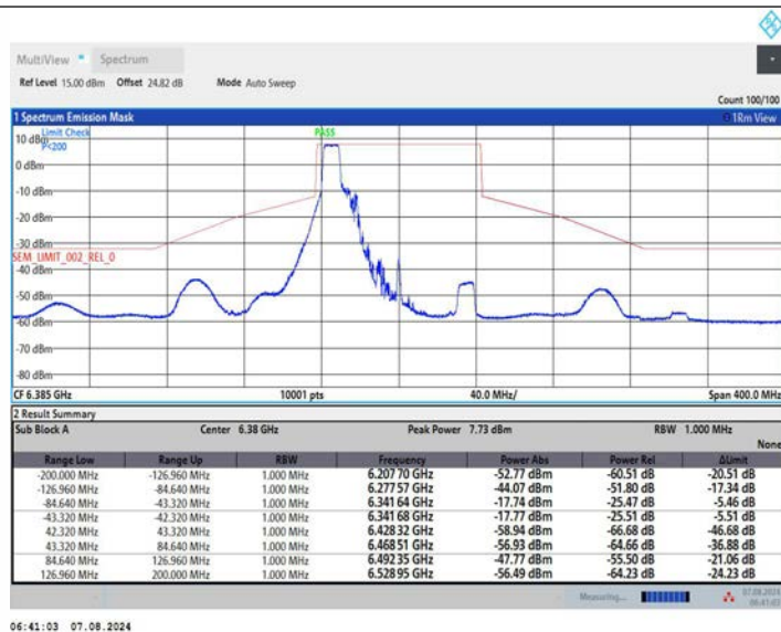
11AX80MIMO_Ant1_6385_242Tone_RU61
