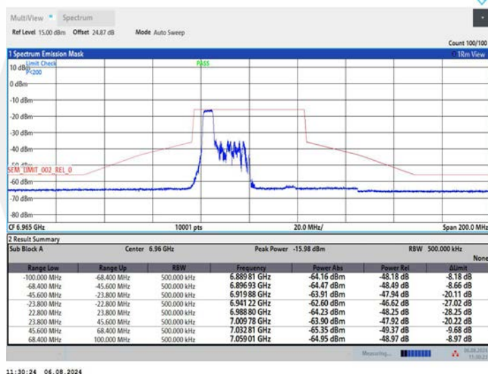
11AX40MIMO_Ant1_6965_106Tone_RU53
