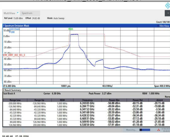
11AX80MIMO_Ant1_6385_484Tone_RU65
