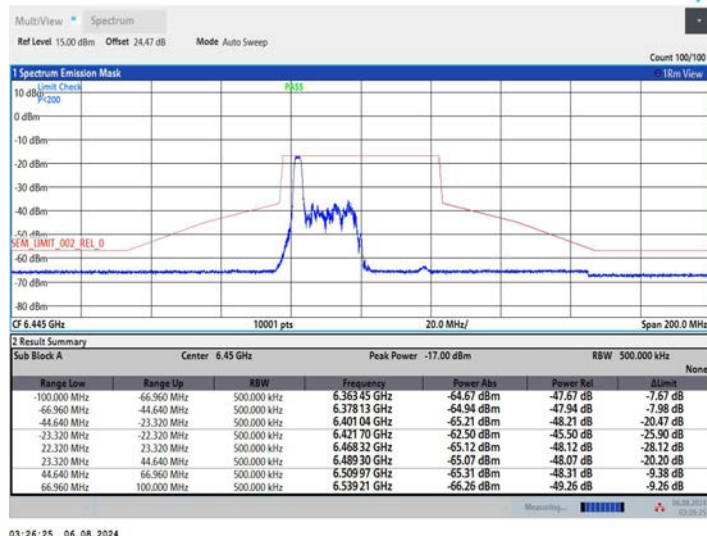
11AX40MIMO_Ant1_6445_52Tone_RU37
