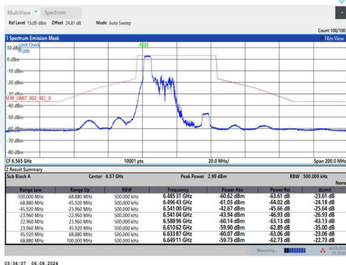
11AX40MIMO_Ant1_6565_106Tone_RU53
