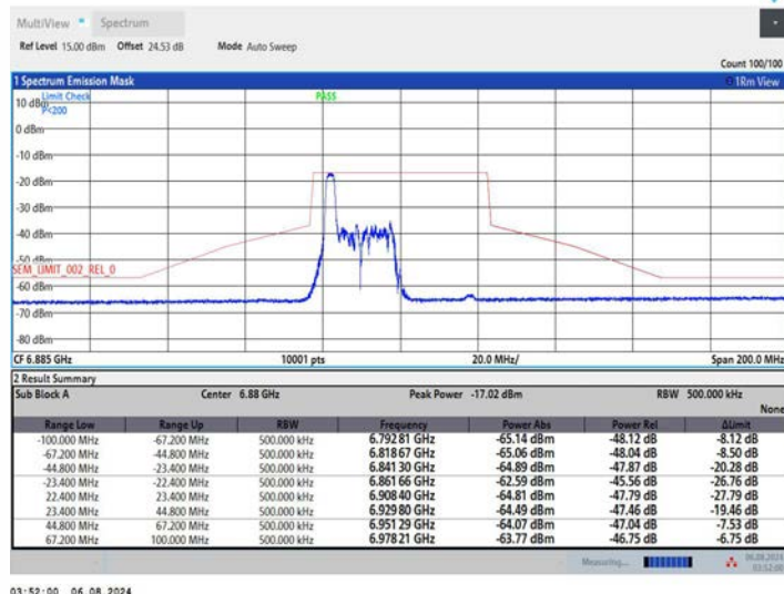
11AX40MIMO_Ant1_6885_52Tone_RU37
