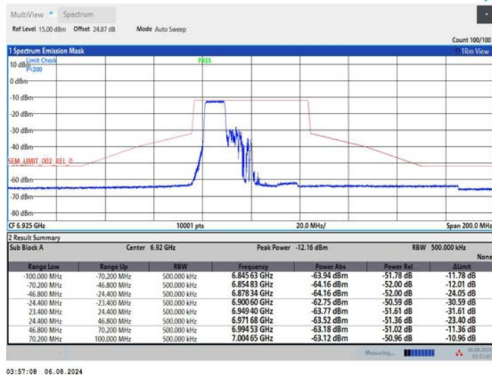
11AX40MIMO_Ant2_6925_242Tone_RU61
