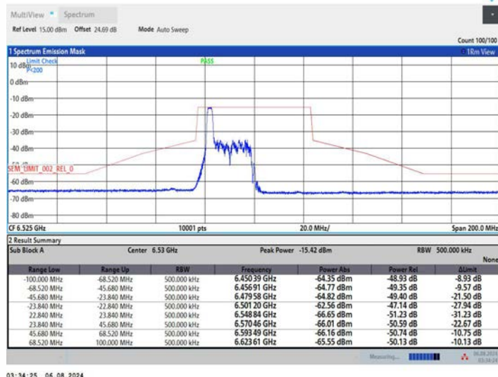
11AX40MIMO_Ant2_6525_52Tone_RU37
