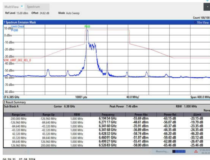
11AX80MIMO_Ant1_6385_52Tone_RU37
