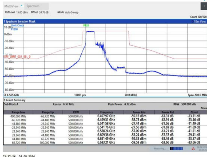
11AX40MIMO_Ant2_6565_242Tone_RU61
