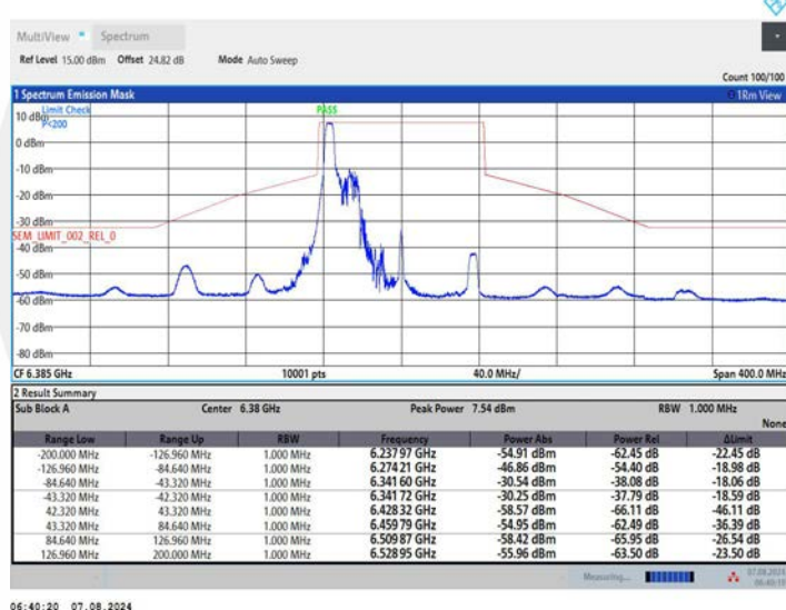
11AX80MIMO_Ant1_6385_106Tone_RU53
