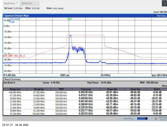
11AX40MIMO_Ant1_6485_52Tone_RU37
