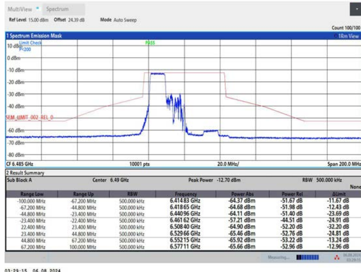
11AX40MIMO_Ant1_6485_242Tone_RU61
