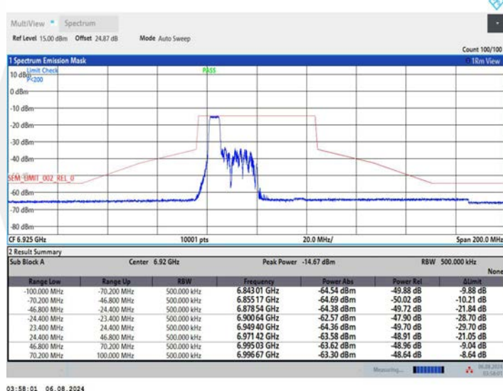
11AX40MIMO_Ant2_6925_106Tone_RU53
