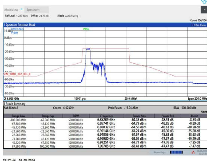
11AX40MIMO_Ant1_6925_106Tone_RU53
