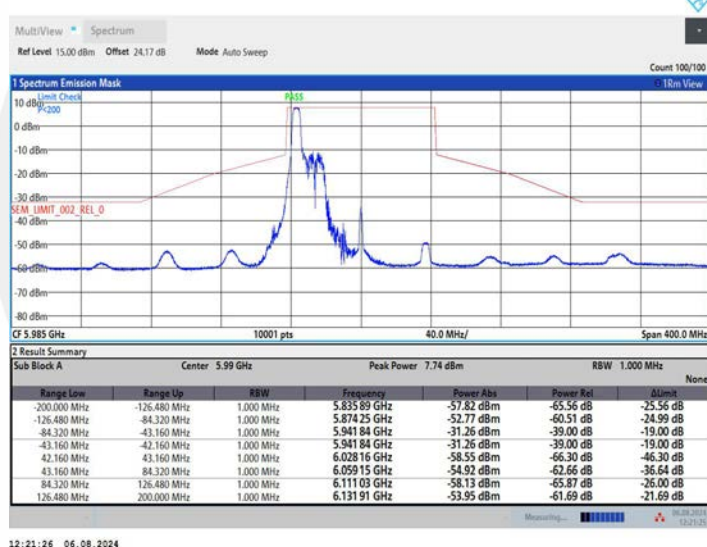
11AX80MIMO_Ant1_5985_106Tone_RU53
