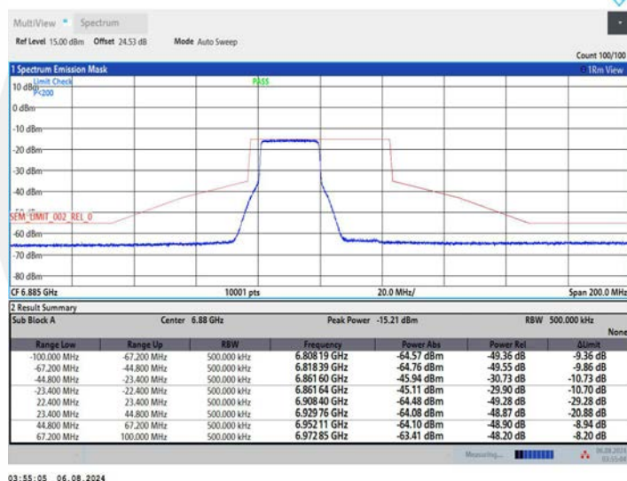
11AX40MIMO_Ant2_6885_26Tone_RU0
