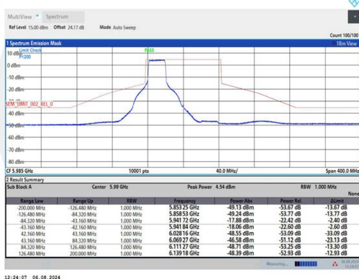
11AX80MIMO_Ant1_5985_484Tone_RU65
