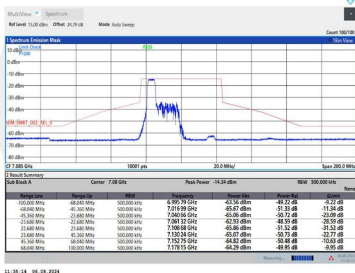
11AX40MIMO_Ant2_7085_106Tone_RU53
