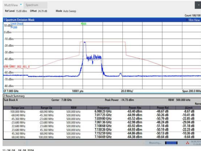
11AX40MIMO_Ant2_7085_52Tone_RU37
