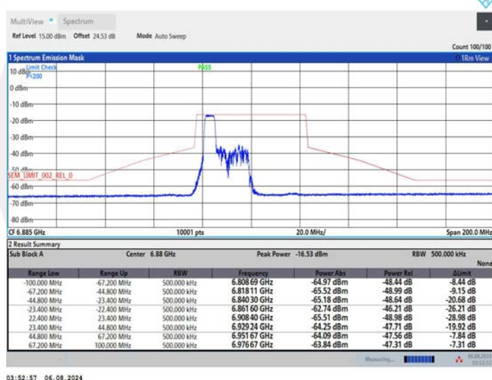
11AX40MIMO_Ant1_6885_106Tone_RU53
