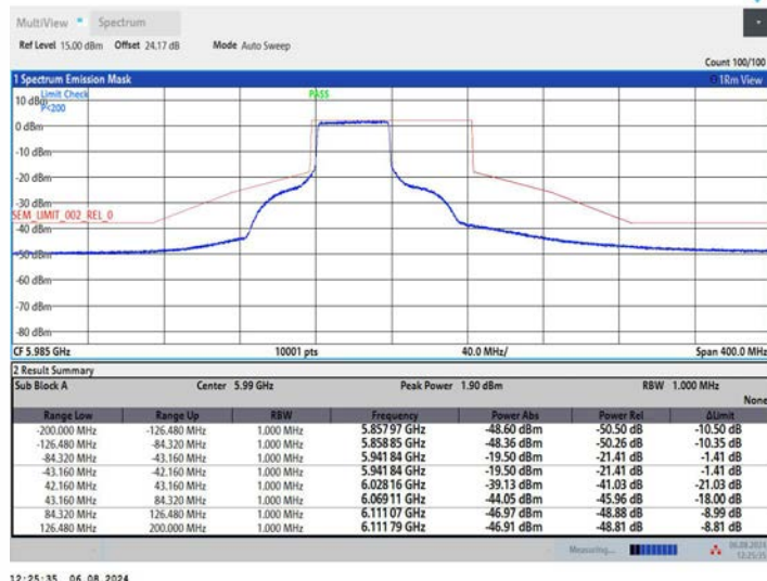
11AX80MIMO_Ant2_5985_26Tone_RU0
