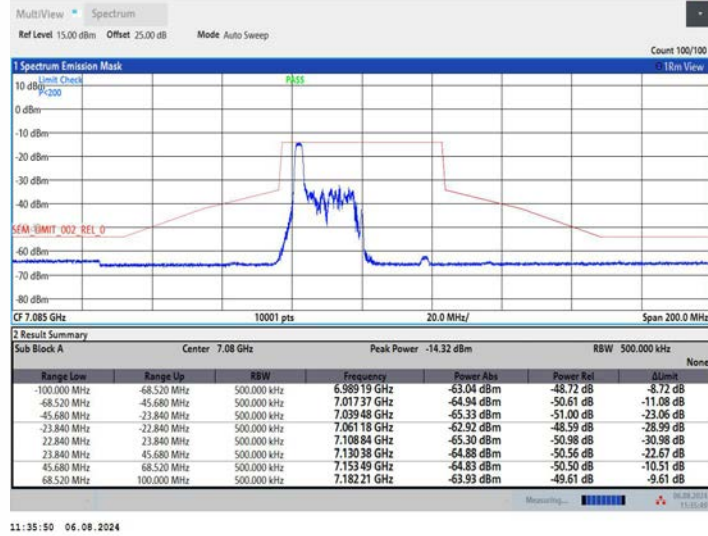
11AX40MIMO_Ant1_7085_52Tone_RU37
