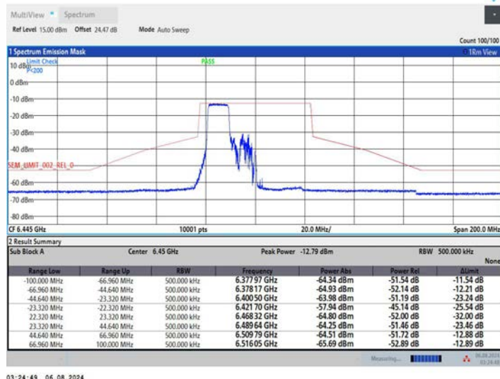
11AX40MIMO_Ant1_6445_242Tone_RU61
