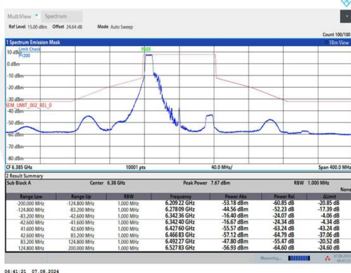
11AX80MIMO_Ant2_6385_242Tone_RU61
