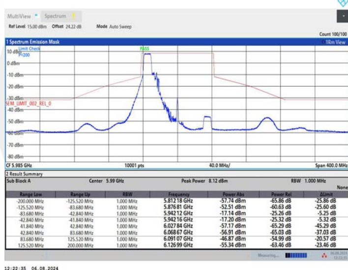
11AX80MIMO_Ant2_5985_242Tone_RU61
