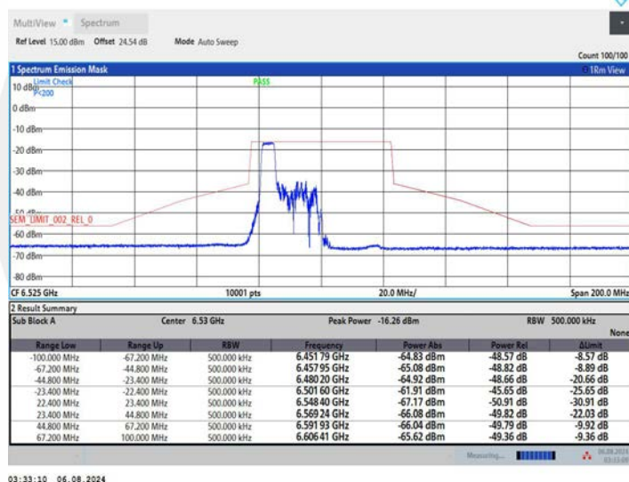
11AX40MIMO_Ant1_6525_106Tone_RU53
