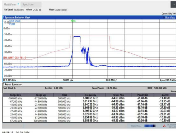
11AX40MIMO_Ant1_6885_242Tone_RU61
