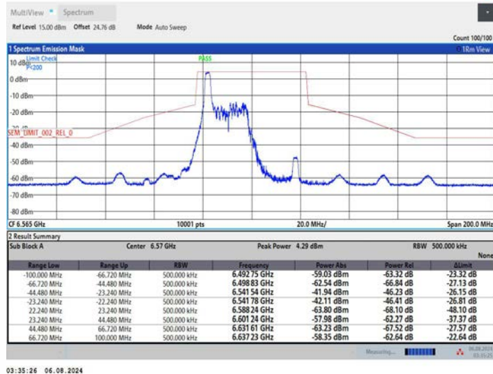
11AX40MIMO_Ant2_6565_52Tone_RU37
