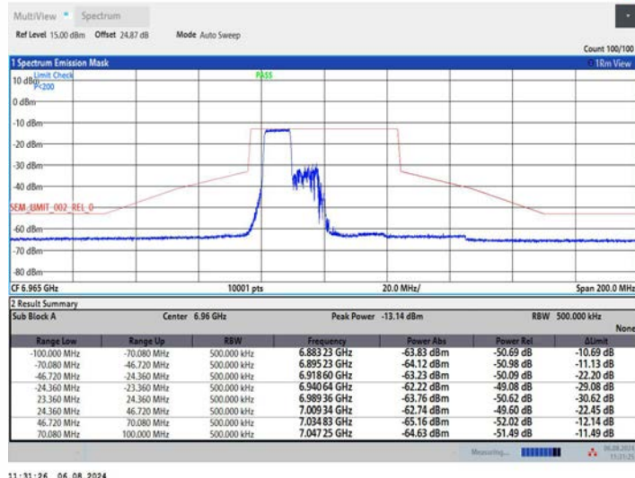
11AX40MIMO_Ant2_6965_242Tone_RU61
