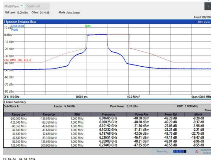
11AX80MIMO_Ant2_6145_26Tone_RU0
