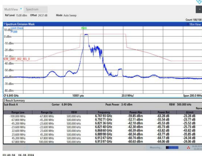
11AX40MIMO_Ant1_6845_106Tone_RU53
