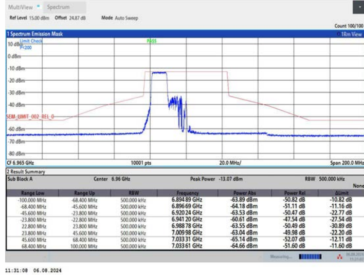
11AX40MIMO_Ant1_6965_242Tone_RU61
