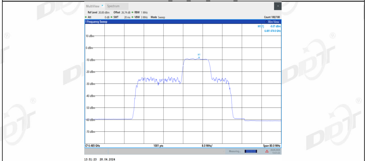
11BE40MIMO_Ant2_6485_106+26_4
