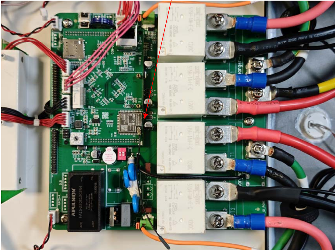
Bluetooth/WiFi Module
