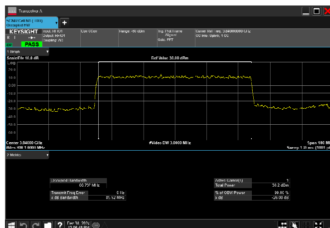
n77_3_90MHz_30kHz_3840MHz_DFT-s-OFDM \pi/2 BPSK_RB243@0
