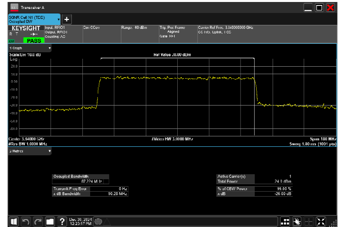
n77_3_100MHz_30kHz_3840MHz_DFT-s-OFDM QPSK_RB270@0
