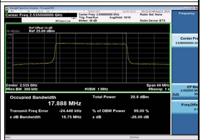
FDD07_MidRange_20_2535_Q16
