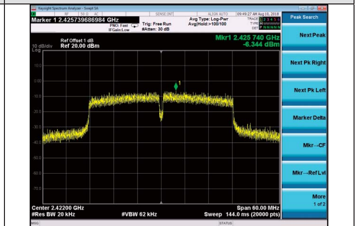
11nHT40-LCH
