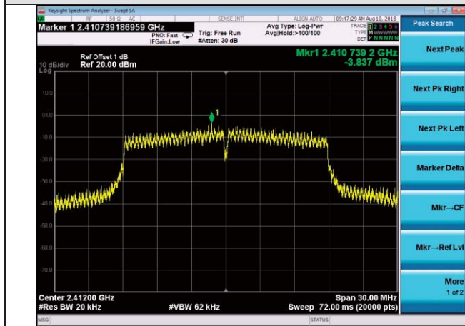
11nHT20-LCH
