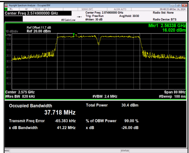
41(2555-2655)-41(2555-2655)-20MHz-20MHz-16QAM-16Q AM-40340-40538-100RB#0-100RB#0-PASS
