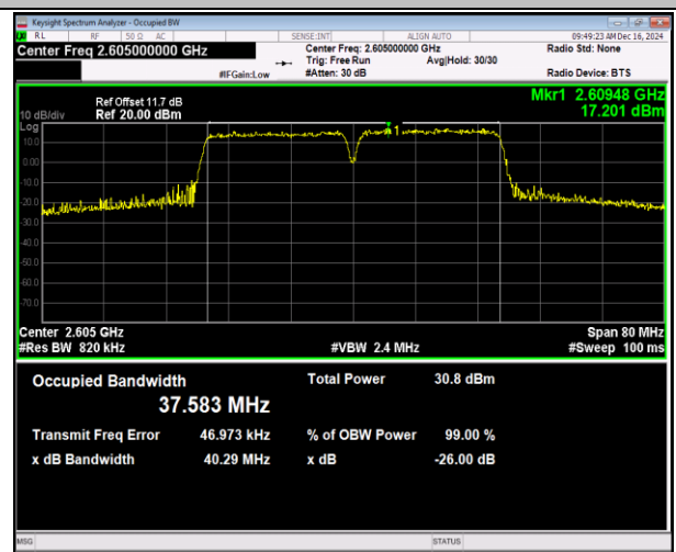
41(2555-2655)-41(2555-2655)-20MHz-20MHz-16QAM-16Q AM-40641-40839-100RB#0-100RB#0-PASS
