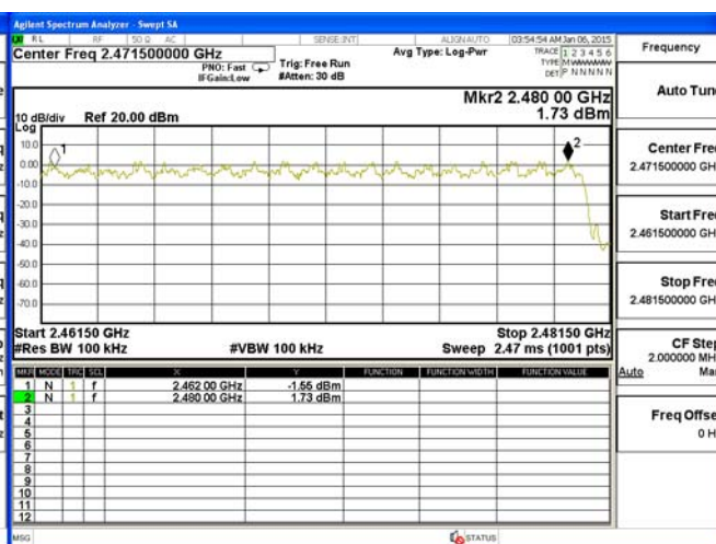
2462-2480MHz
