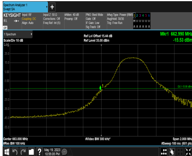
Band71-5MHz-QPSK-133147-1RB#24
