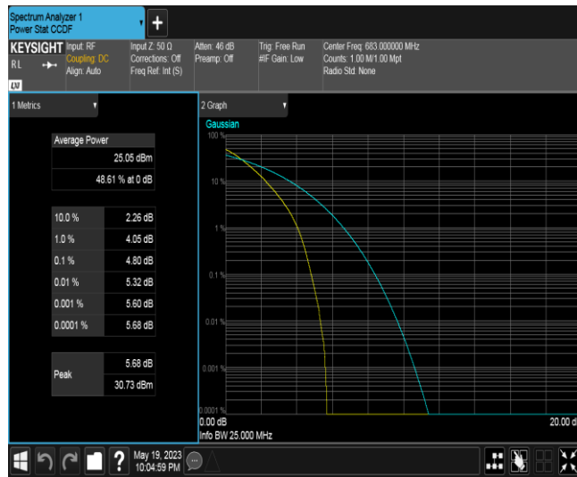
Band71-20MHz-QPSK-133372-1RB#0
