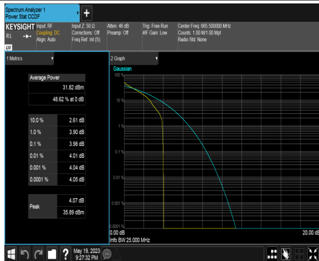
Band71-5MHz-QPSK-133147-25RB#0
