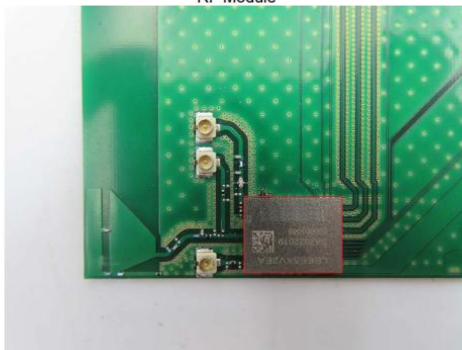
RF Module
