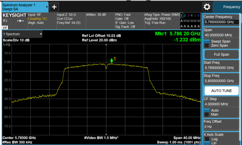
11AC20MIMO_Ant2_5785
