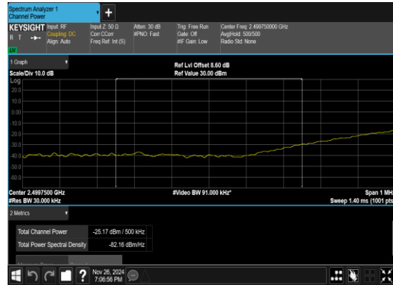
N7(25M)_DFT-s-OFDM_BPSK Edge_1RB_Left_Low_CH_CHP_PASS
