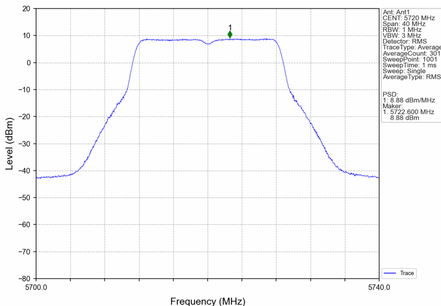
802.11a_HCH_5720MHz_Ant1_NTNV
