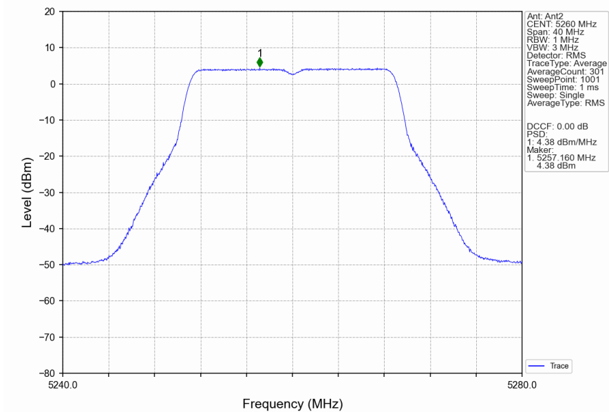
802.11n(HT20)_LCH_5260MHz_Ant2_NTNV
