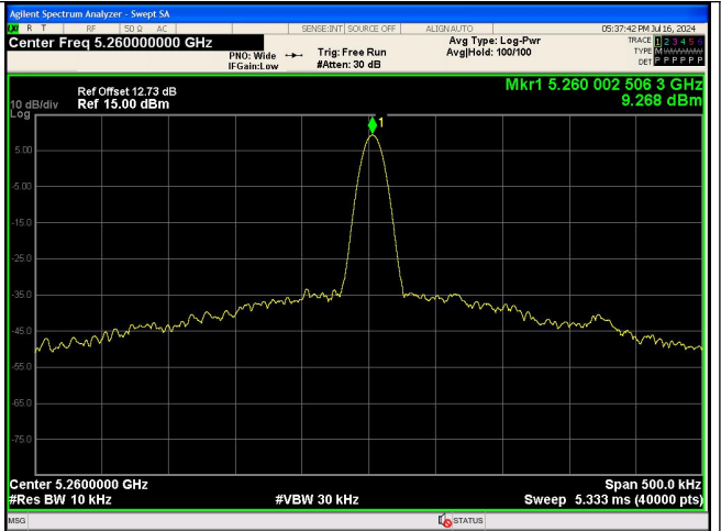
NT/NV_Antenna 0 IEEE 802.11n_Channel 52_20MHz
