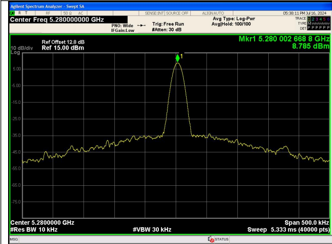
NT/NV_Antenna 0 IEEE 802.11n_Channel 56_20MHz
