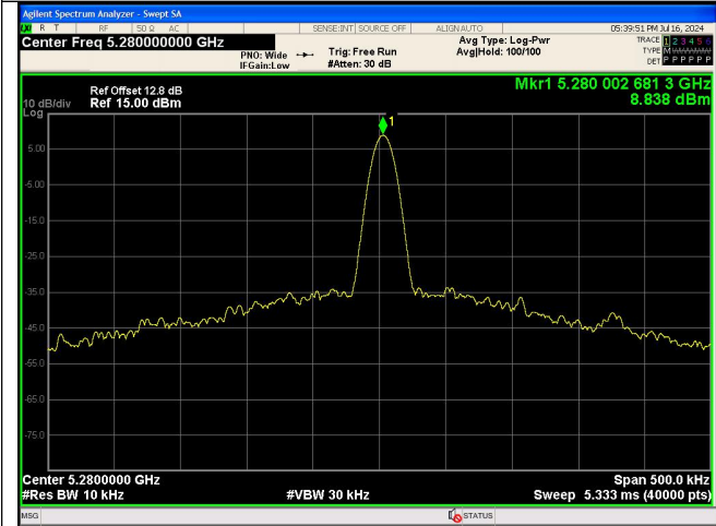
NT/NV_Antenna 0 IEEE 802.11ac_Channel 56_20MHz
