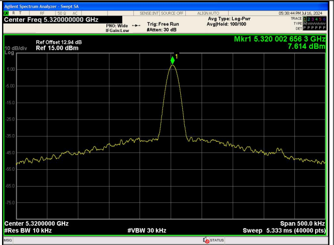
NT/NV_Antenna 0 IEEE 802.11n_Channel 64_20MHz
