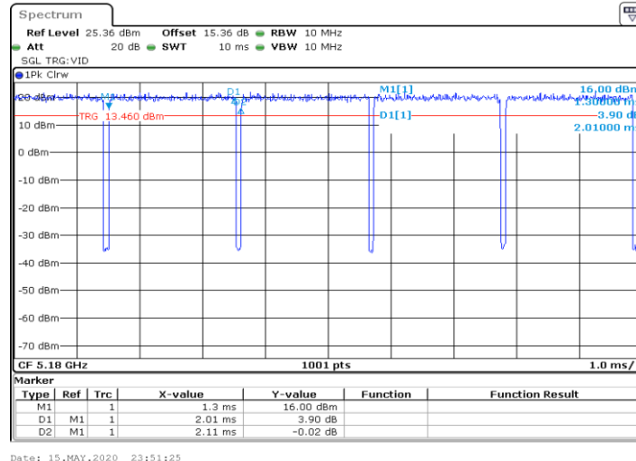
11A-MIMO_Ant2_5180
