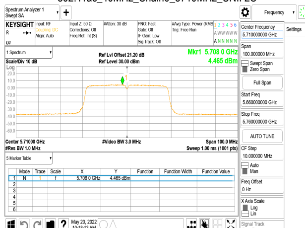
802.11ac_40MHz_Chain0_5710MHz_UNII 3
