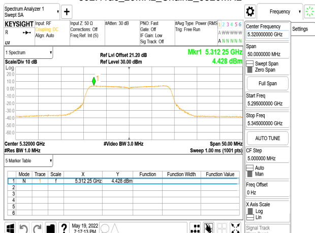
802.11ac_20MHz_Chain2_5320MHz
