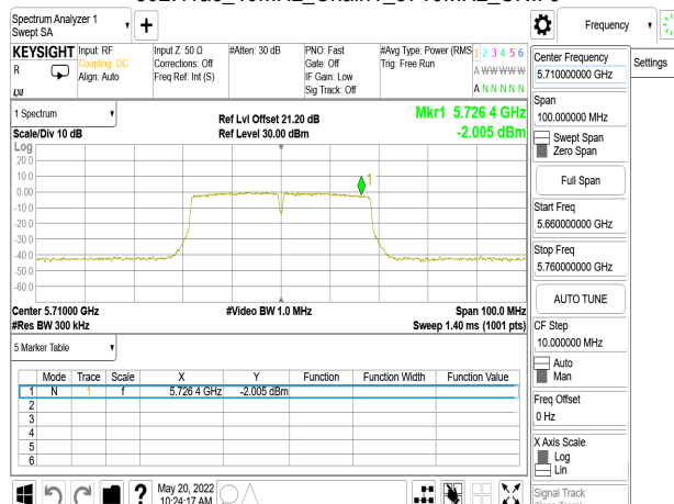
802.11ac_40MHz_Chain1_5710MHz_UNII 3
