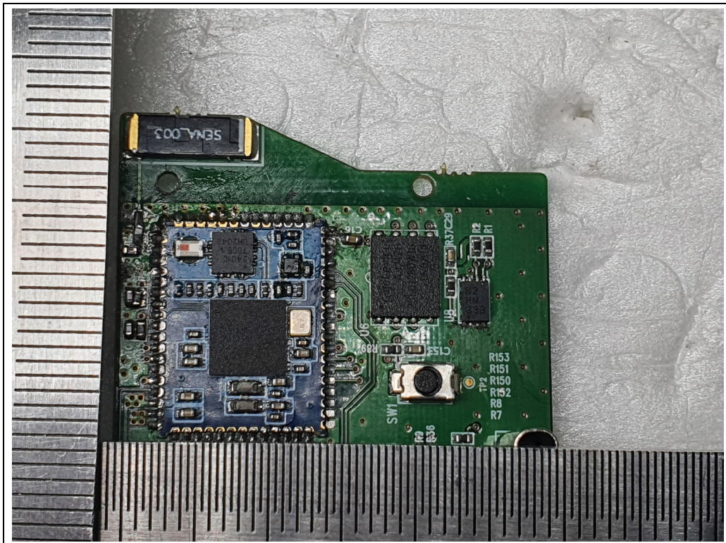
<Module&Antenna>
