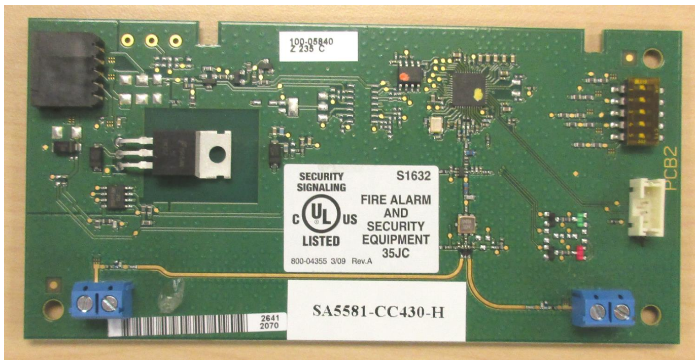
PCB BOTTOM
