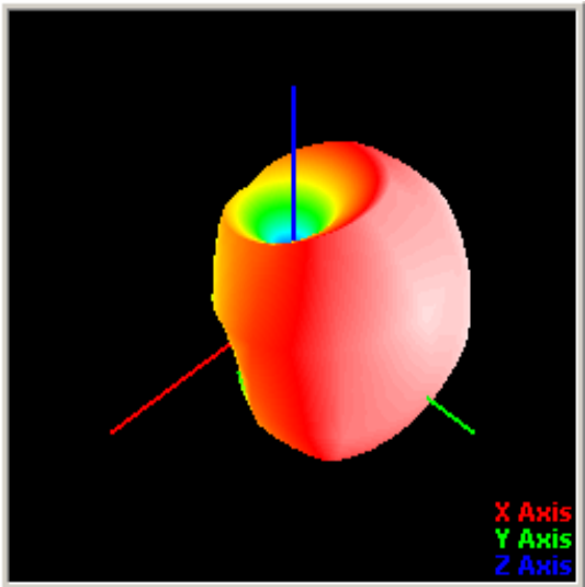
天线方向图
