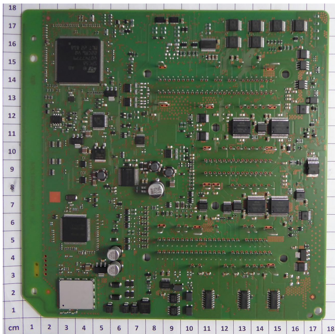
PCB bottom
