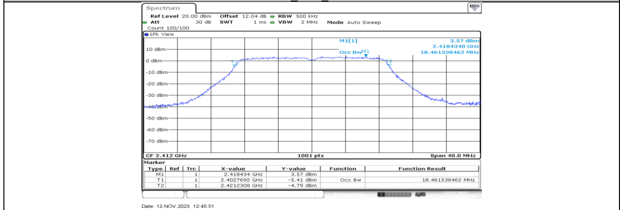
11N20MIMO Ant0 2412
