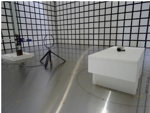
9 kHz - 30 MHz
