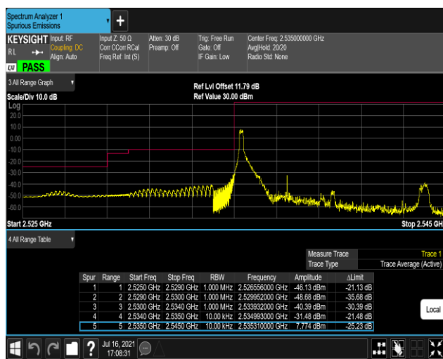
Band41-5MHz-QPSK-40065-25RB#0
