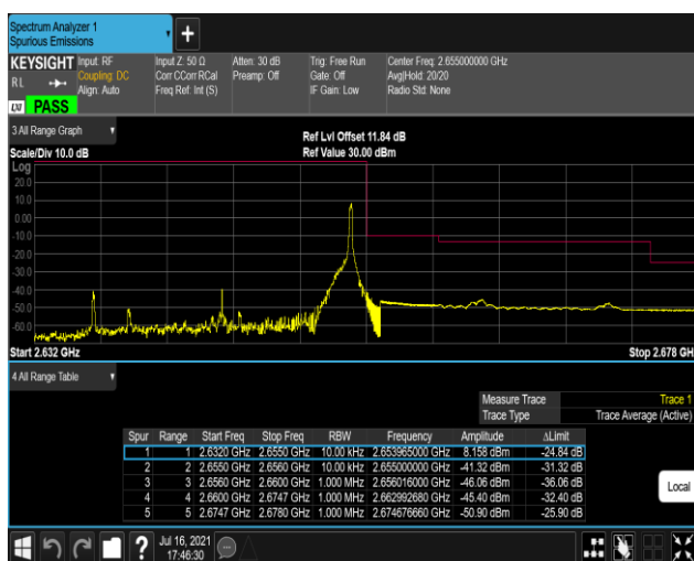
Band41-20MHz-QPSK-41140-1RB#99
