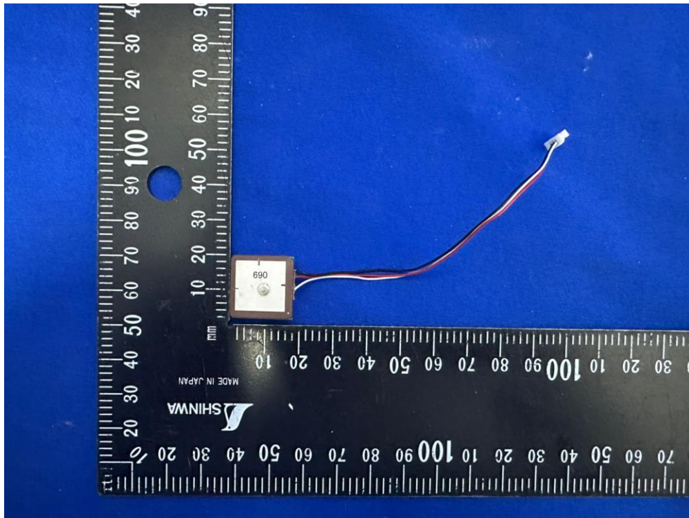
(19) EUT Photo (GPS module)
