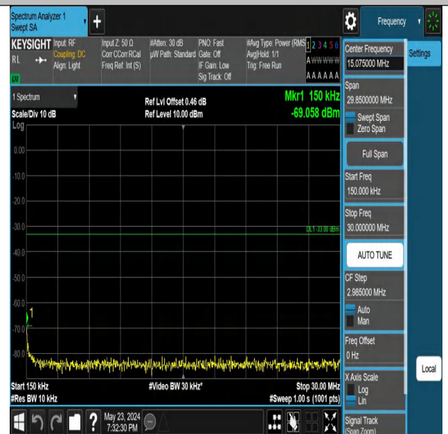
Band66 20MHz QPSK 132572 1RB#0 0.15~30 0.15~30
