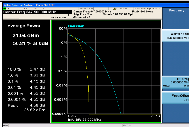
Band5-3MHz-QPSK-20635-1RB#0
