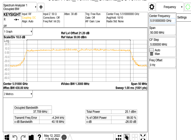
802.11ax_40MHz_Chain2_5510MHz
