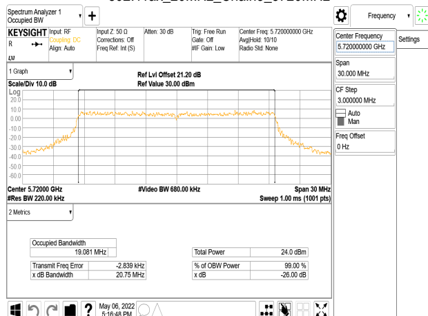
802.11ax_20MHz_Chain3_5720MHz
