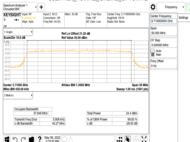
802.11ax_40MHz_Chain2_5710MHz
