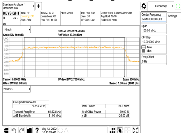
802.11ax_80MHz_Chain0_5610MHz
