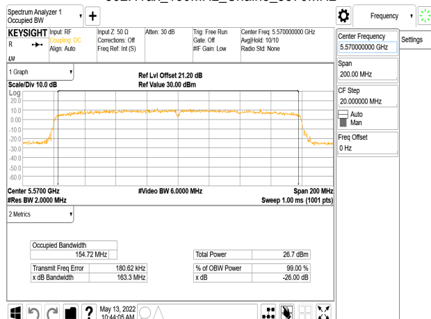
802.11ax_160MHz_Chain3_5570MHz
