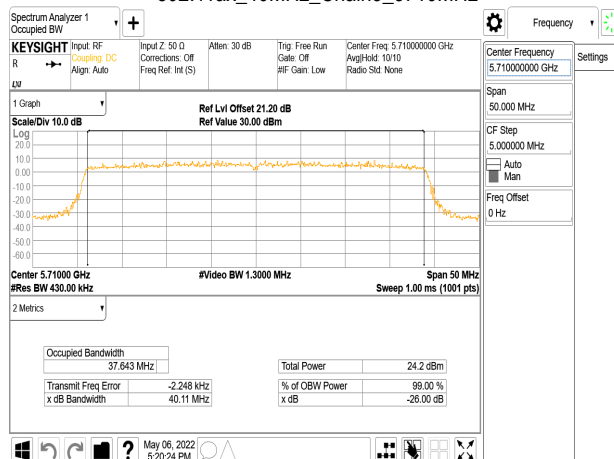
802.11ax_40MHz_Chain3_5710MHz
