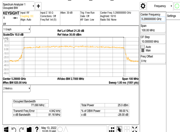
802.11ax_80MHz_Chain2_5290MHz
