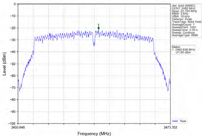
802.11n(HT20)_HCH_2462MHz_Ant2 (MIMO)_NTNV
