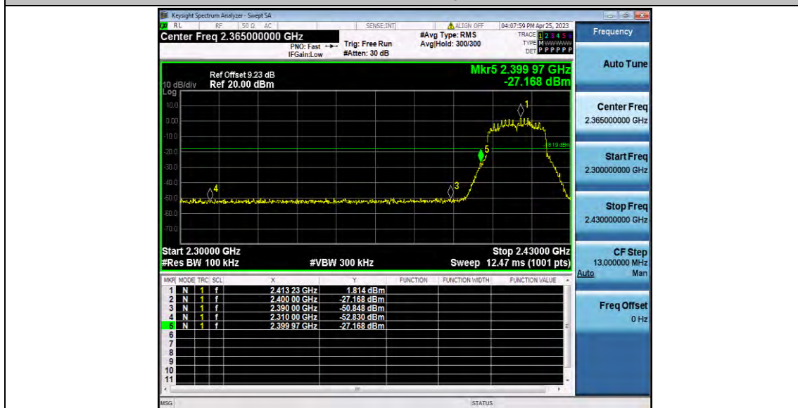
11AX20SISO_Ant2_Low_2412
