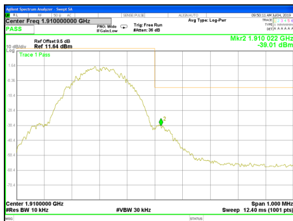
GPRS_1900_Higher_Band edge
