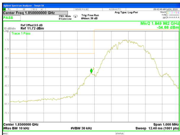
GPRS_1900_Lower_Band edge
