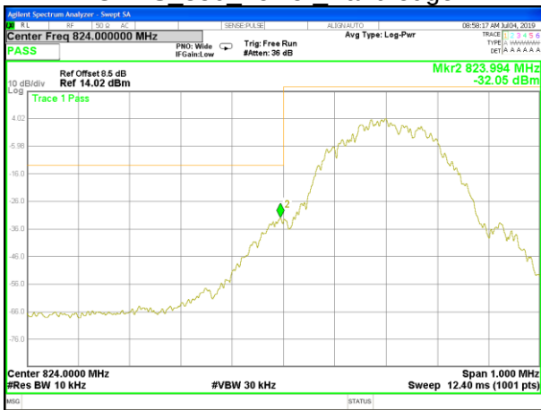
EGPRS_850_Lower_Band edge
