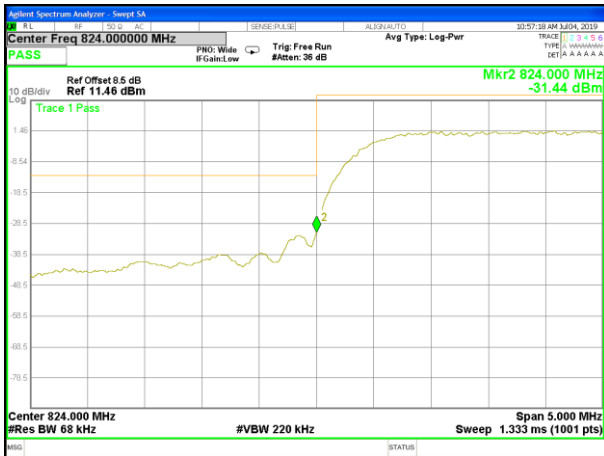
B5_WCDMA_Lower_Band edge
