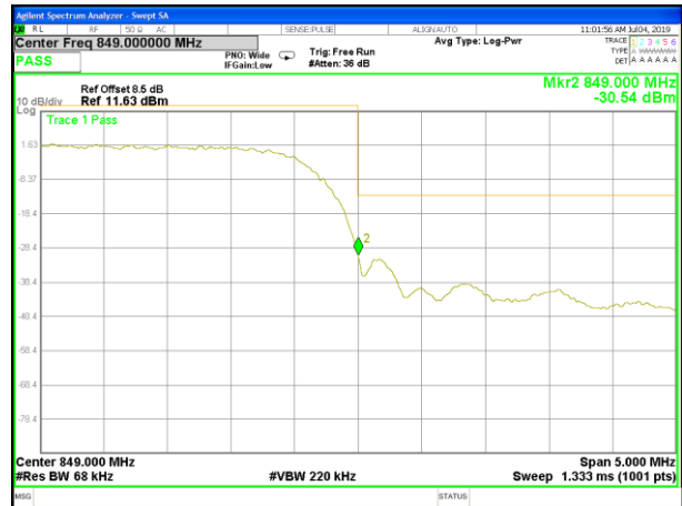
B5_WCDMA_Higher_Band edge
