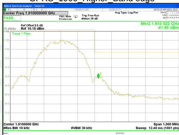
EGPRS_1900_Higher_Band edge
