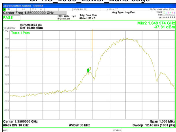
EGPRS_1900_Lower_Band edge
