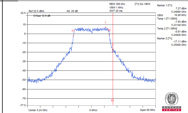
802.11a_Chain 3 / CH48
