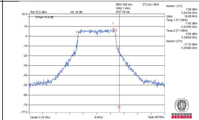
802.11a_Chain 5 / CH48
