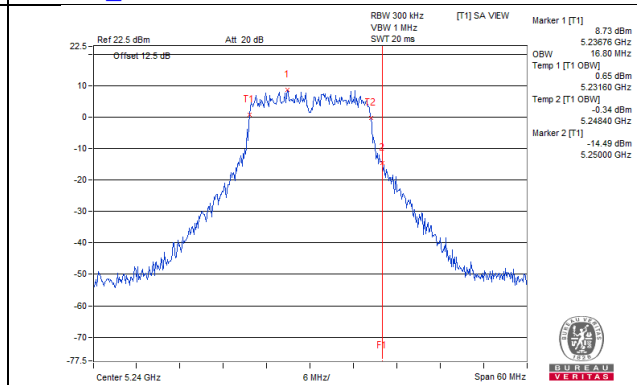
802.11a_Chain 7 / CH48
