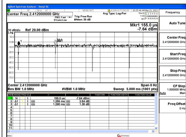
802.11n (20 MHz)
