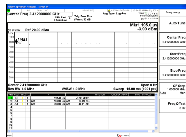
802.11n (20 MHz)
