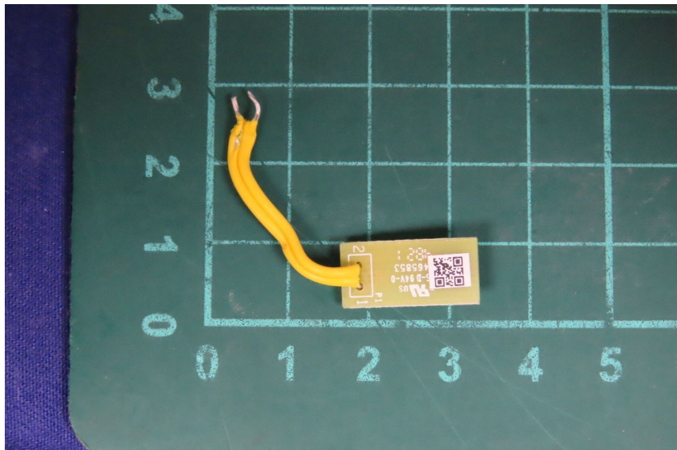
(16) EUT Photo
