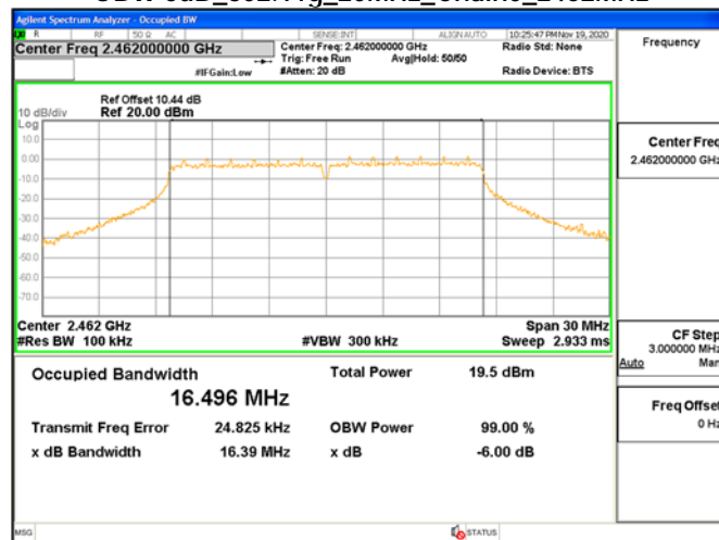
OBW 6dB_802.11g_20MHz_Chain0_2462MHz
