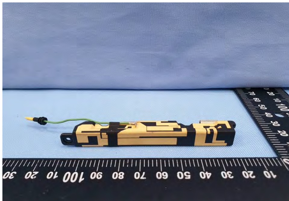
EUT Photo (86)
