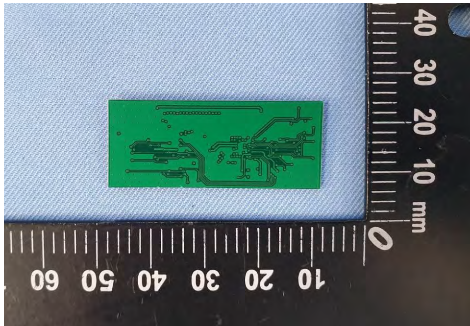
EUT Photo (96)
