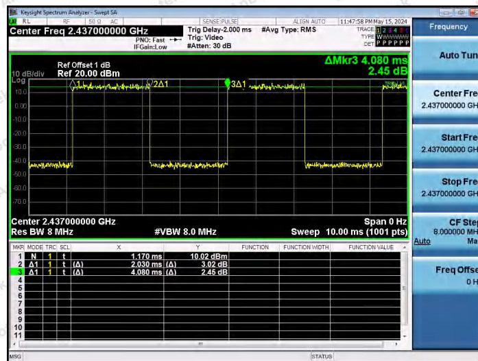
NTNV-11G-Ant1-2437
