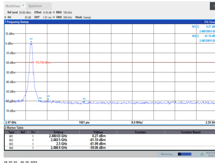
BLE 1M_Ant0_High_2480
